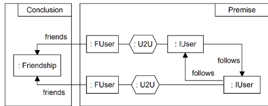
Fig. 3. EnforceFriendship
