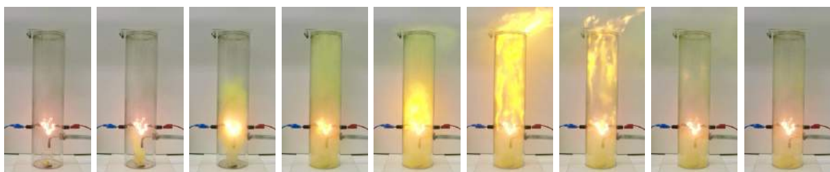
Abbildung 20: Aufwirbelung und Entzündung im Bereich der Geschwindigkeitsreduzierung (Bildsequenz aus einem Video).
