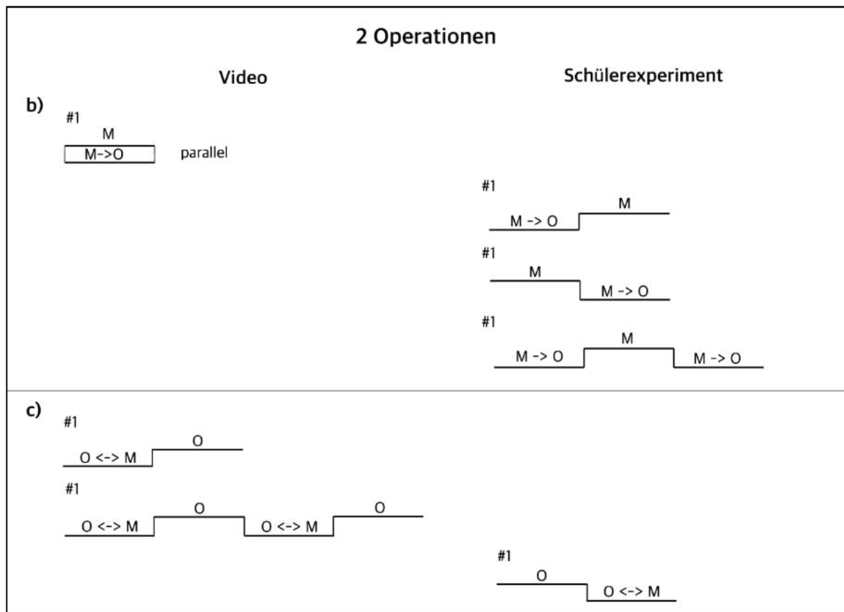
Abbildung 58: Denkwege mit zwei Analogieoperationen ( Beschreibung und abbildende Beschreibung ) differenziert nach der Präsentationsform des Modellexperiments und deren absoluter Häufigkeit.
