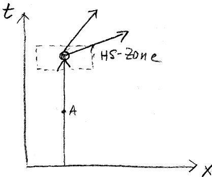
Skizze 6: Darstellung der seelischen Raumzeit als Koordinatensystem
