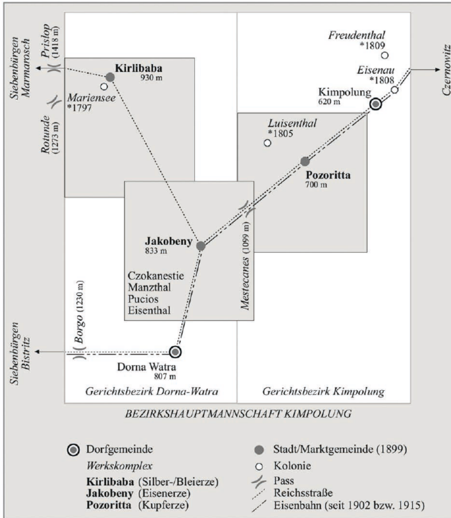
Abb. 66: Struktur und Lage des Bergbaugesbietes Jakobeny vor dem Ersten Weltkrieg. Höhenangaben nach Spezialkarte der Österreichisch-Ungarischen Monarchie (Normalnull Triest).
