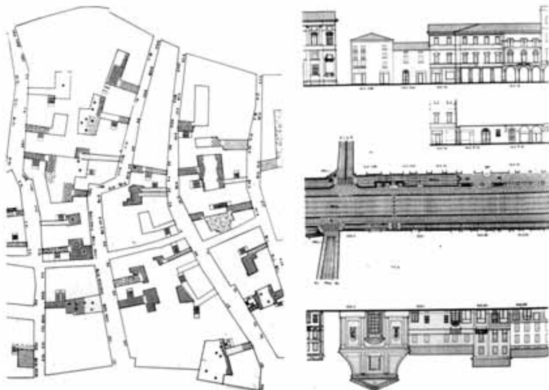
7.5 – Esempio di lettura tematica: vuoti e pieni
