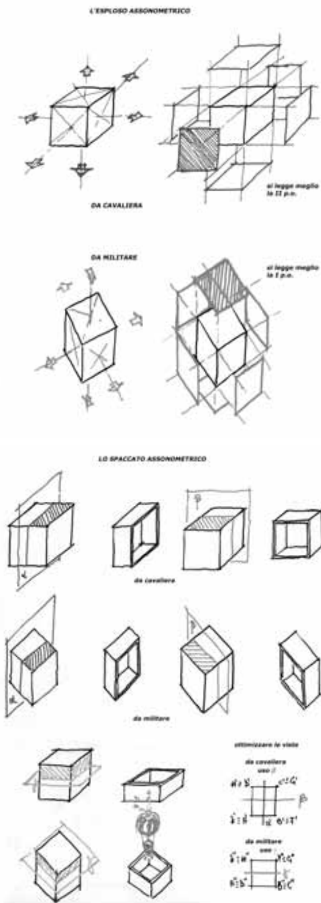
3.6 - L'esploso e lo spaccato assometrico: operazioni fondamentali
