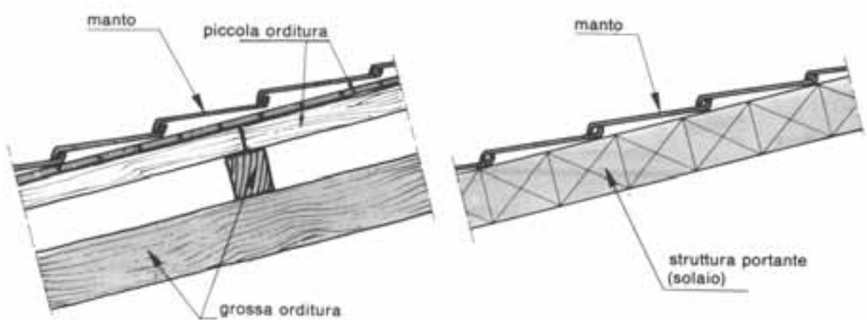
4.23 – Dettagli costruttivi
