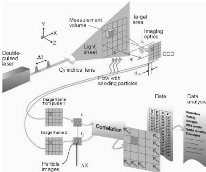
Fig. 57: La catena di misura con tecnica PIV
