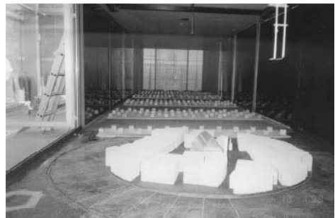
Fig. 33 Foto del modello Palazzo della Ragione in Padova alloggiato in camera di prova della galleria del vento
