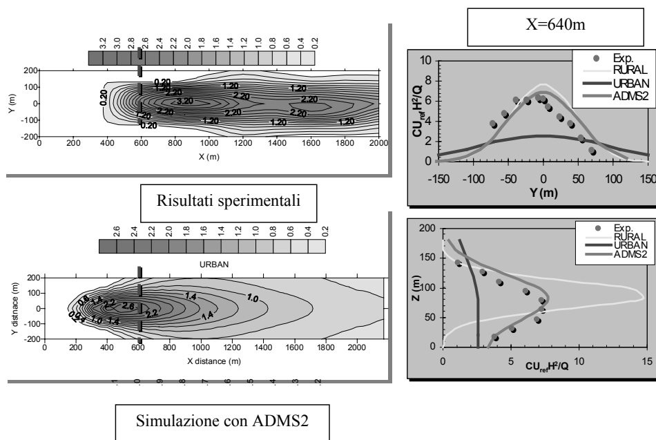
Fig. 48 Schemi di diffusione degli'inquinanti ottenuti analizzando i risultati delle prove in galleria del vento
