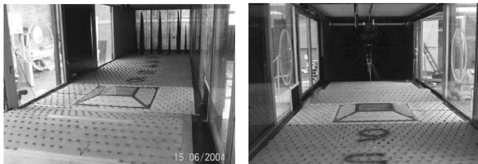
Fig. 51 Foto del modello della discarica utilizzato nelle prove in galleria del vento
