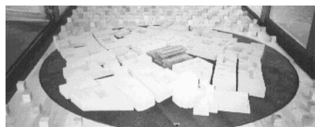
Fig. 27 Foto del modello della copertura posta all'interno della galleria del vento
