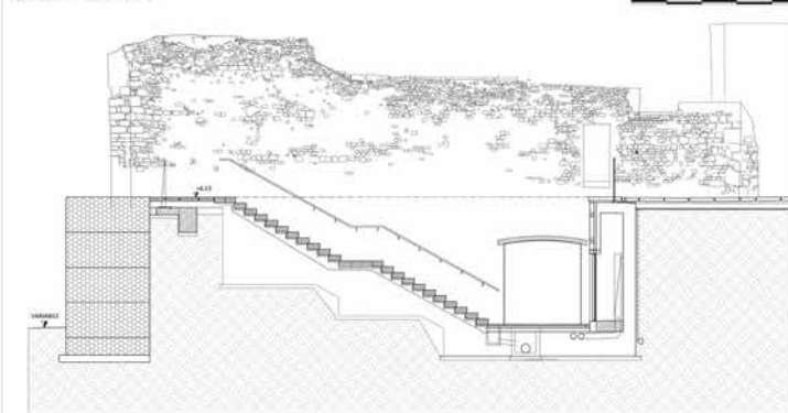
PROGETTO - SEZIONE C-C'
