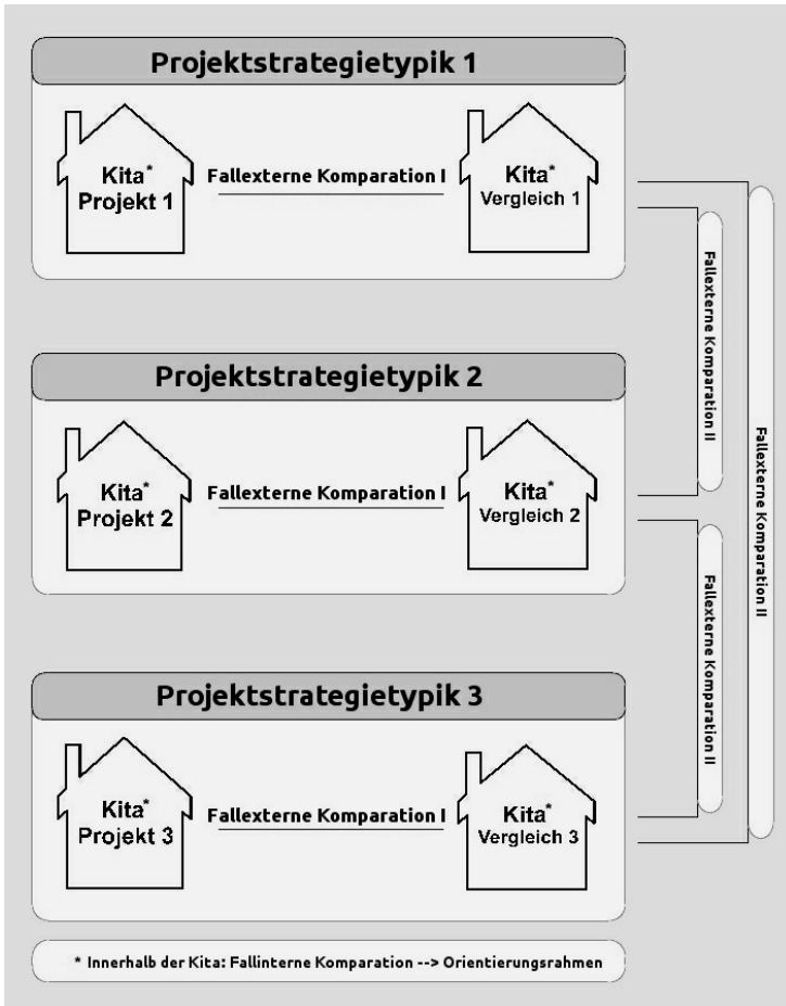
Abbildung 1: Komparatives Auswertungsvorgehen
