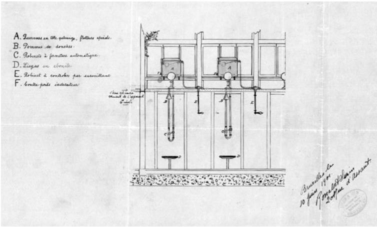
Figure 35. Pavillon de bains-douches de la place du Jeu de balle. Robinet de contrôle, 1901 (AVB, Plan portefeuille 3141)
