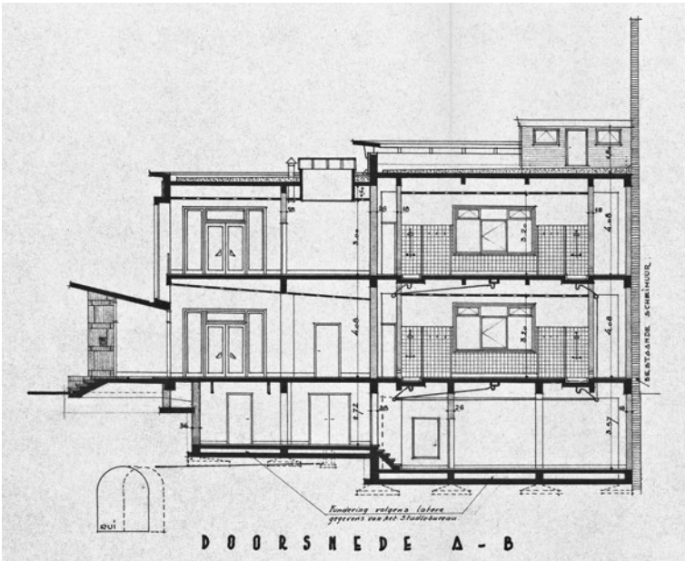
Figure 11. Bains publics de la Zakstraat, 1958 (AVA, 672#317)
