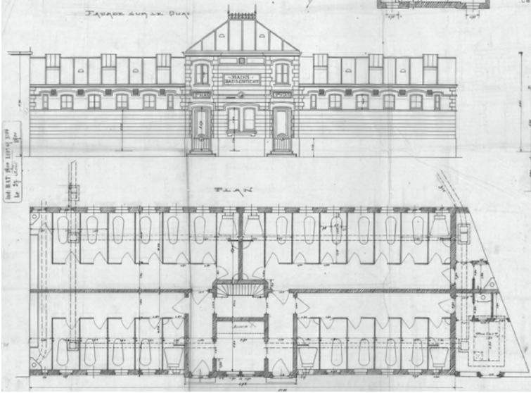
Figure 24. Bains publics du Bijlokekaai. Façade et plan du rez-de-chaussée, 1900 (AVG, G12/1900/Q/14)
