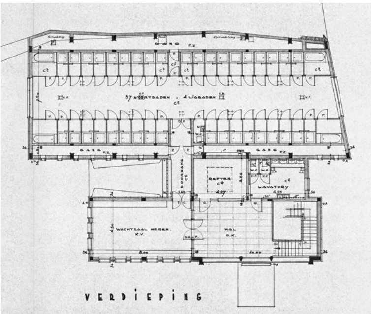
Figure 12. Bains publics de la Zakstraat. Plan du premier étage, service des hommes, 1958 (AVA, 672#317)
