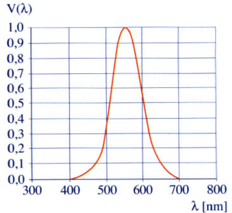
Courbe photopique de l'œil humain
