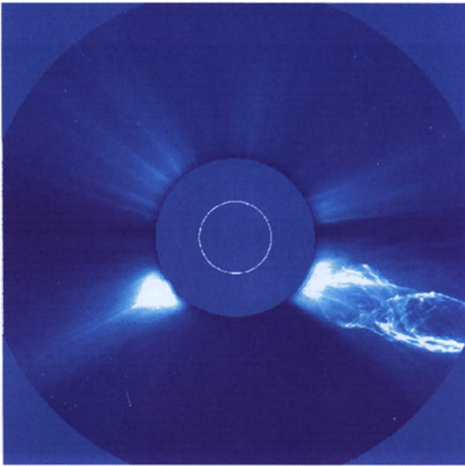
Figure 1.39 - A droite de l'image, une éjection de masse coronale (ce jour-là associée à une éruption solaire)
