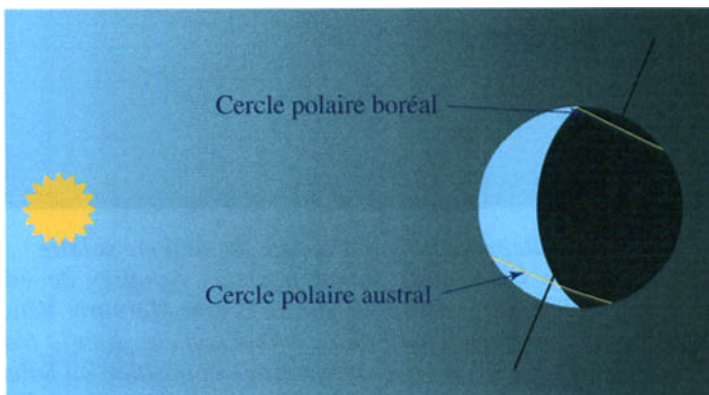
Figure 2.4 - Les cercles polaires pendant l'hiver boréal
