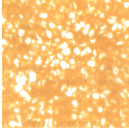
Figure 1.7 - Cette image de la granulation solaire a été prise le 20 juin 1999, avec THEMIS, Télescope Héliographique pour l'Etude du Magnétisme et des Instabilités Solaires, l'un des très grands équipements du CNRS, développé en collaboration avec l'Italie Elle représente un carré d'environ 24 000 kilomètres de côté. (crédit THEMIS/CNRS/INSU/CNR)
