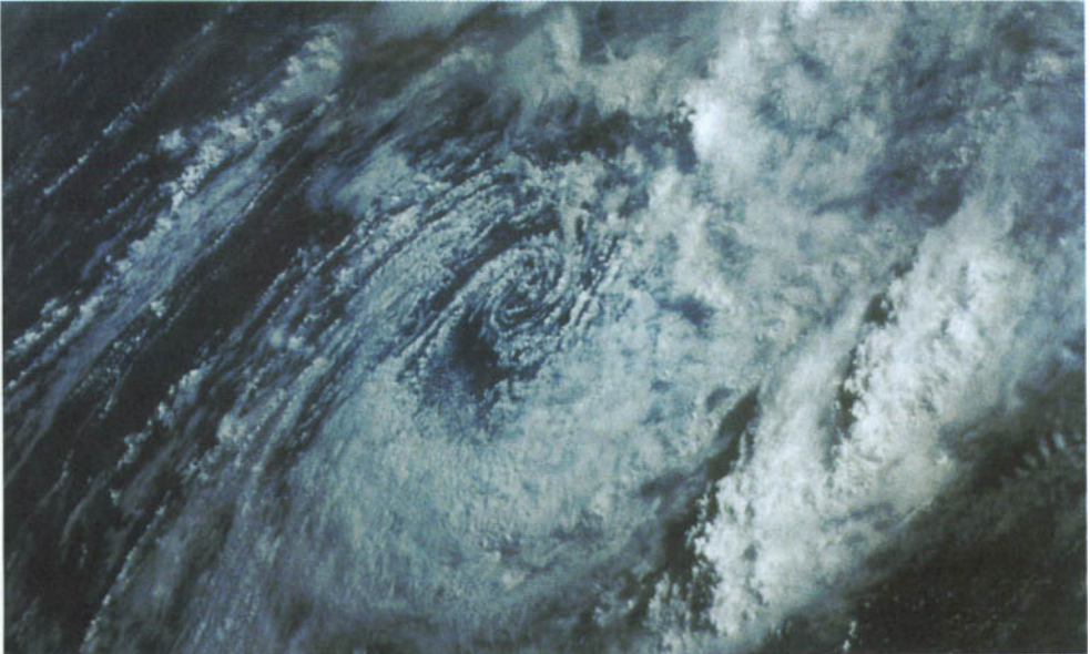
Figure 2.9 - La troposphère correspond à la zone de l'atmosphère objet de la météorologie classique
