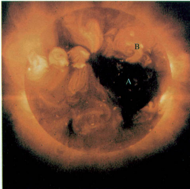
Figure 1.33 - Le Soleil photographié par le satellite YOHKOH en rayons X, le 5 décembre 1999
