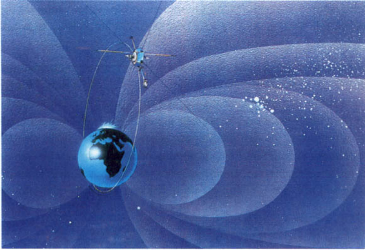
Figure 2.5 - Vue d'artiste des lignes de champ magnétique autour de la Terre Le satellite suédois, Viking, avait pour mission l'observation de l'environnement de la Terre. Il a été lancé en février 1986 (crédit Viking, Agence suédoise de l'Espace).
