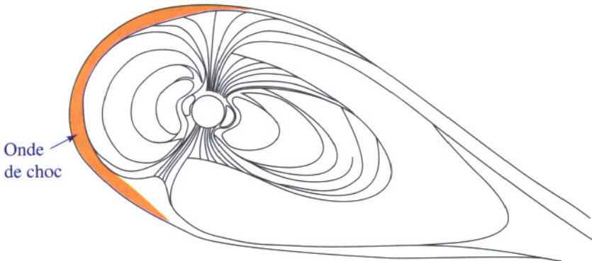
Figure 2.17 - En amont de la Terre, l'onde de choc (ici en orange) crée un échauffement du vent solaire. Celui-ci s'accélère avant de longer la magnétopause.
