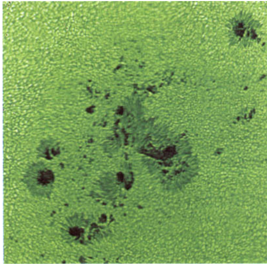
Figure 1.21 - Photographie de taches solaires dans la chromosphère observée dans la raie alpha de l'hydrogène (656,28 nanomètres) le 14 juillet 2000, enregistrée au Dunn's Solar Telescope du National Solar Observatory/Sacramento Peak Observatory
