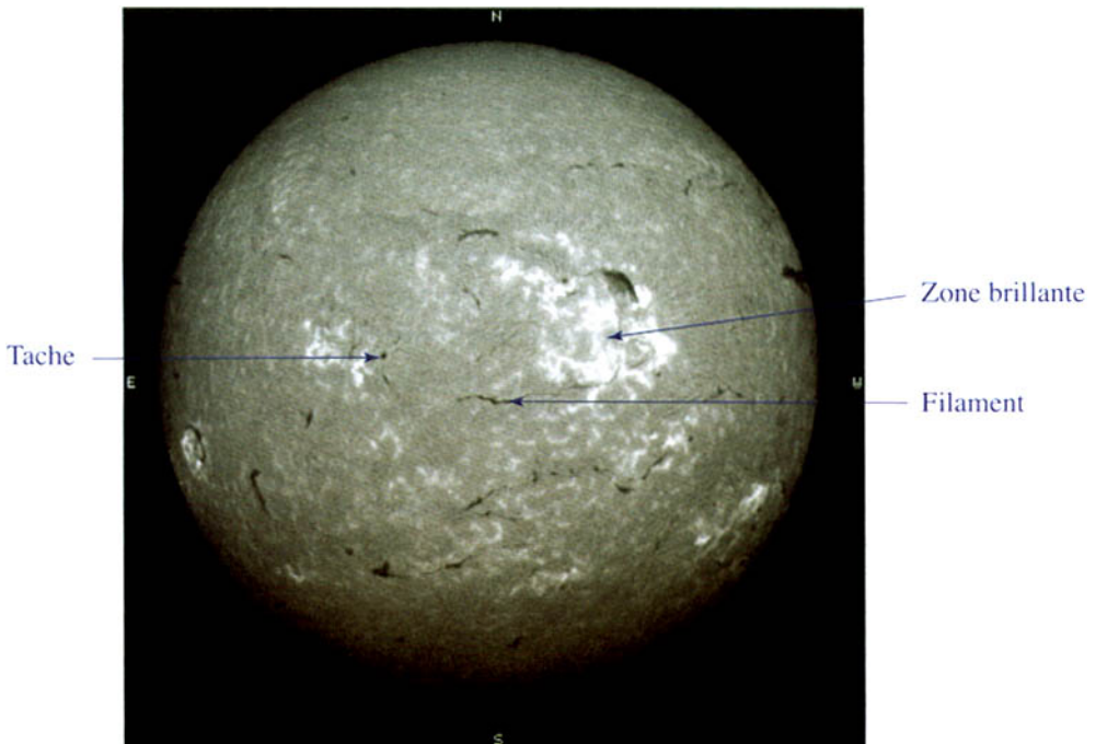
Figure 1.27 - Image de la photosphère, le 5 novembre 2000 (en période active), par le spectrohéliographe de Meudon en H\alpha (656,3 nanomètres) On y voit de nombreux filaments, des taches solaires, des zones brillantes. (crédit DASOP, Observatoire de Paris-Meudon ; CNRS)
