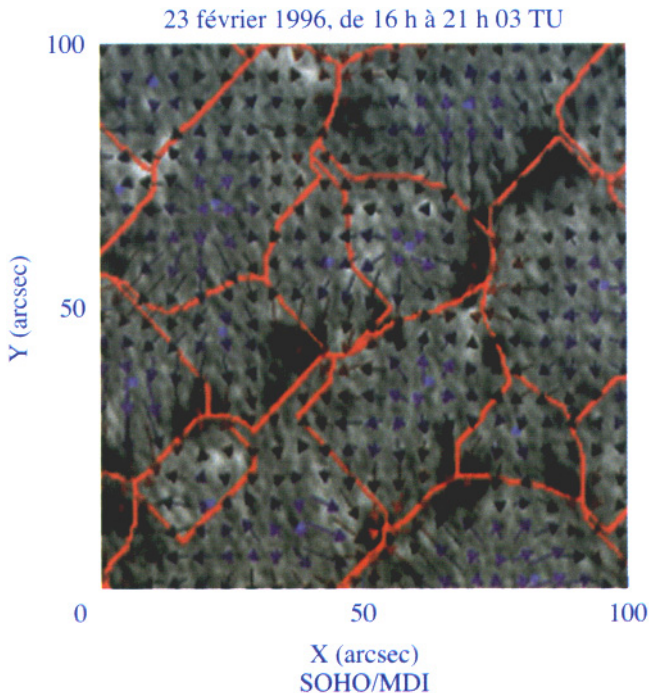
Figure 1.8 - Réseau de supergranulation superposé en rouge sur une photographie de l'instrument MDI à bord de SOHO Les flèches représentent la vitesse ascensionnelle des supergranules, le bleu allant vers le haut. Le côté de l'image représente environ 120 000 kilomètres.
