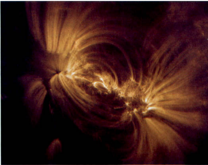
Figure 1.25 - Le satellite TRACE visualise les boucles magnétiques au-dessus de la photosphère
