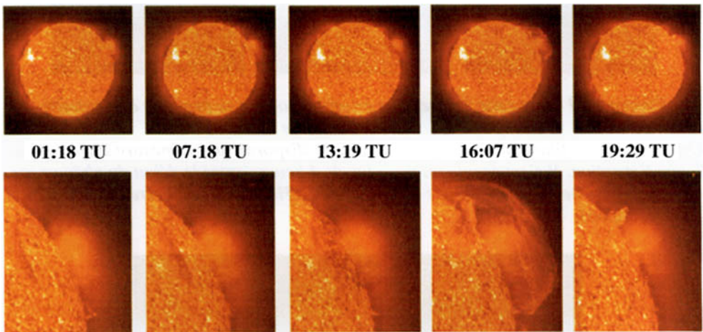
Figure 1.31 - Voici une spectaculaire séquence d'images, prise par SOHO-EIT le 27 août 1997, montrant une belle éruption solaire
