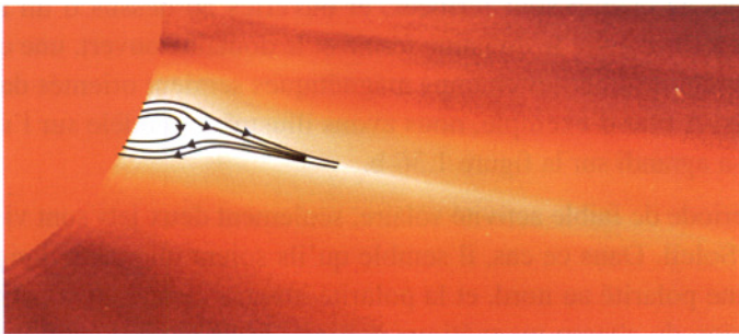
Figure 1.36-b - Illustration du modèle de jets. Les lignes représentent les lignes de champ magnétique, et les flèches la direction de ce champ.
