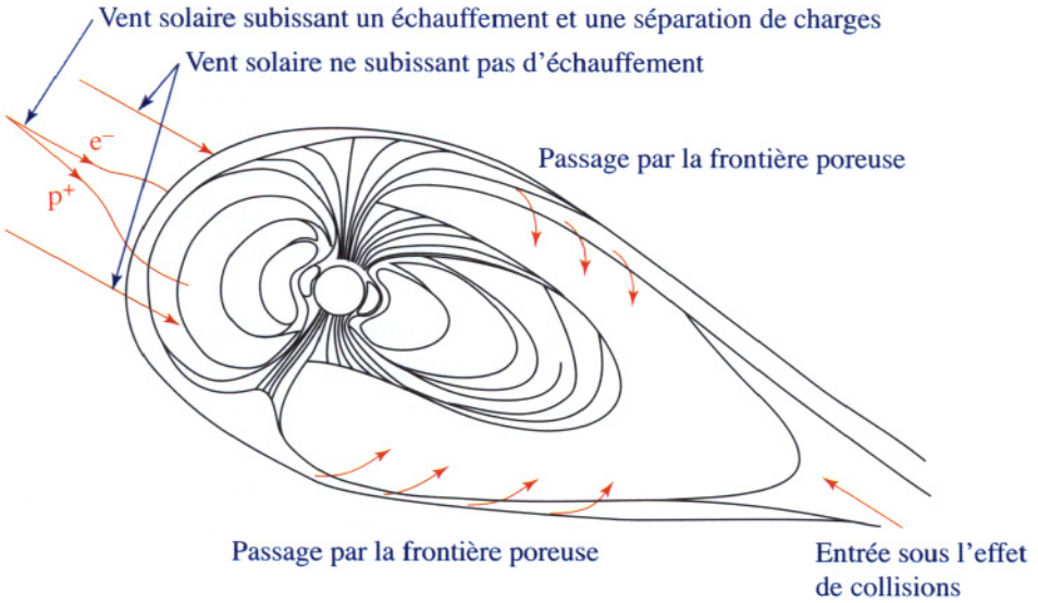
Figure 2.18 - Entrées de particules du vent solaire dans la magnétosphère
