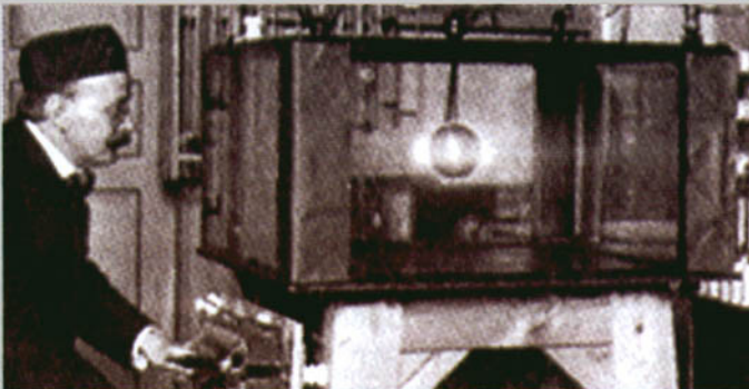
Figure 2.24 - BIRKELAND devant sa Terrella
