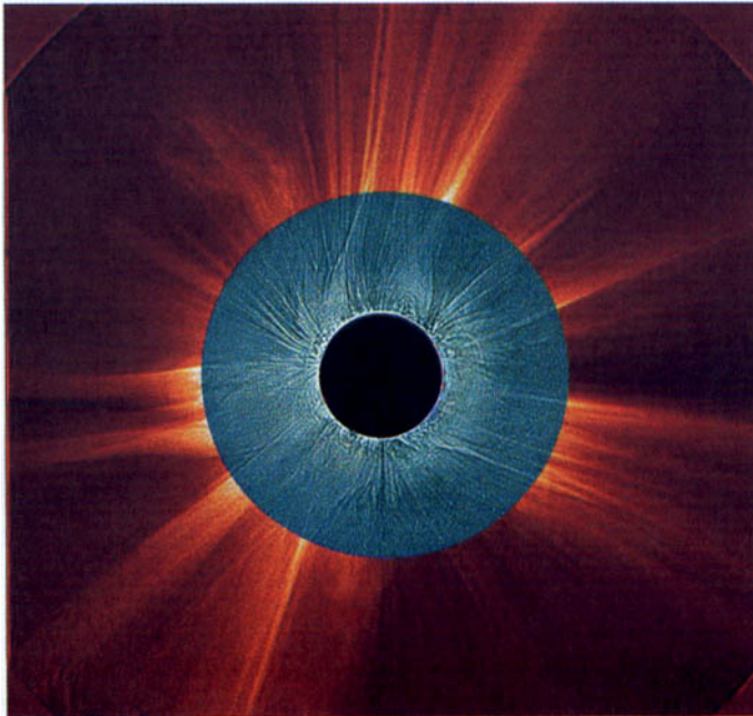
Figure 1.43 - Montage des différentes couches atmosphériques du Soleil, montrant la structure magnétique à diverses échelles, le 11 août 1999, lors de l'éclipse totale (crédit S. Koutchmy, IAP-CNRS, LASCO/SOHO)
