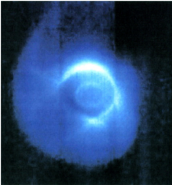
Figure 2.33 - Photographie (en fausses couleurs) de l'environnement de plasma de la Terre lors d'un orage magnétique. Le satellite survole la Terre au-dessus du pôle Nord. On distingue nettement l'ovale auroral dont le rayonnement est intensifié. La sphère plus blanche représente la position et la taille de la Terre. Le Soleil se trouve vers le coin en haut à droite de l'image (crédit NASA, Groupe scientifique du satellite IMAGE).
