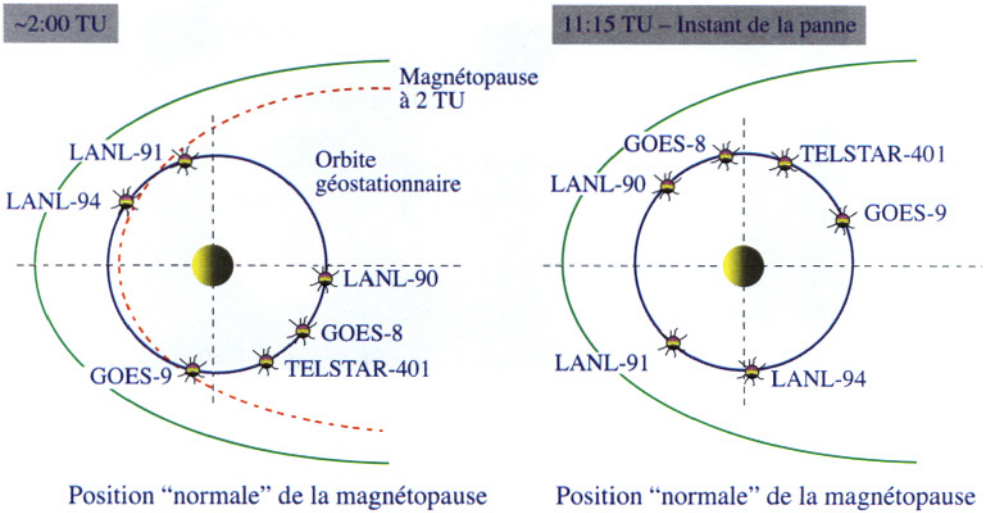
Figure 3.24 - Position des satellites géostationnaires (sur le cercle bleu) La position normale de la magnétopause est figurée en vert. Sa position supposée est montrée sur la figure de gauche, en rouge, à 2 heures (Temps Universel). A droite, on voit où se trouvait le satellite TELSTAR au moment de sa perte.
