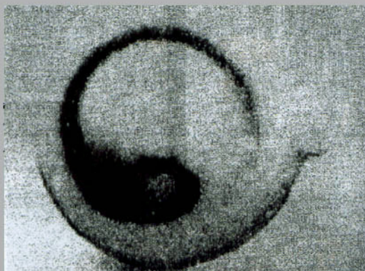
Figure 2.25 - Reconstitution de l'ovale auroral par BIRKELAND
