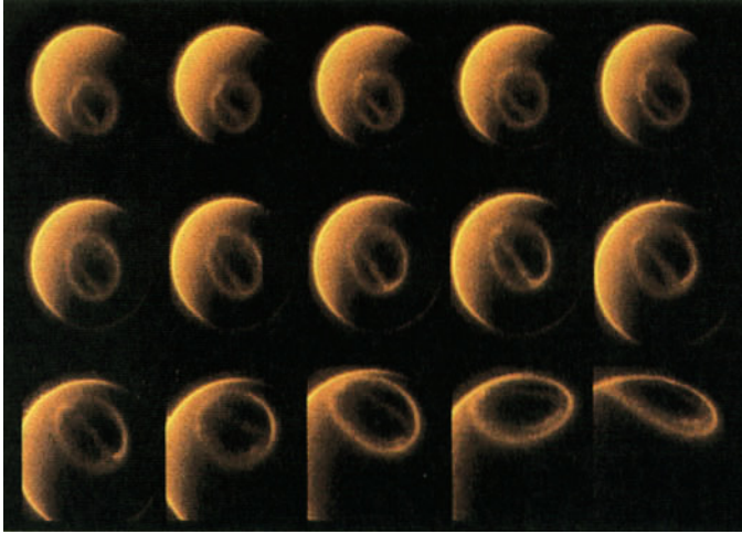
Figure 2.32 - Sur cette photographie de Dynamics Explorer, on voit une séquence de croissance puis de décroissance d'un arc Théta, le 8 novembre 1981, commençant à 14:12 TU et terminant à 17:02 TU. L'apparent grossissement de la Terre vient de l'orbite du satellite qui s'en rapproche (crédit NASA).
