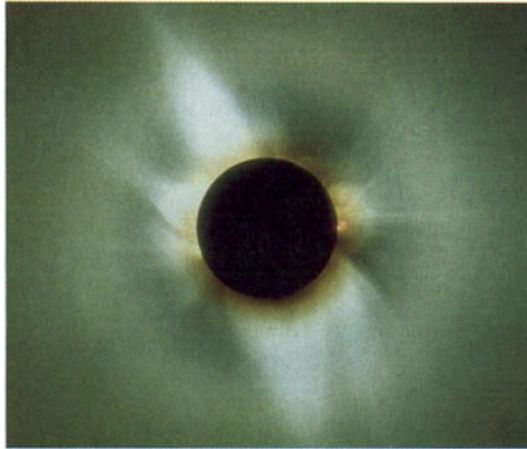
Figure 1.28 - On distingue une protubérance de région active sur le bord du disque solaire, photographiée en lumière blanche lors de l'éclipse totale de Soleil du 11 juillet 1991 depuis Mauna Kea à Hawaïi (crédit S. Koutchmy, IAP-CNRS)
