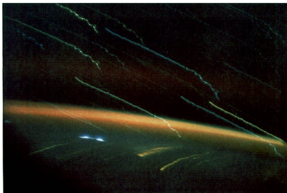
Figure 2.14 - Emission de la raie rouge vers 250 kilomètres d'altitude, photographiée depuis la station soviétique Saliout 6 en 1978. Les traits bleus et blancs sont les étoiles qui semblent défilier pendant la prise de vue. En bas, le limbe de la Terre (crédit S. Koutchmy, IAP-CNRS).
