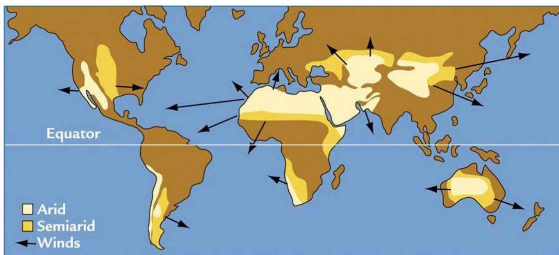
Figure 6. Le dernier maximum glaciaire : expansion des zones désertiques, des calottes glaciaires des Laurentides en Amérique du Nord et scandinave en Eurasie, et réduction des zones tropicales en Afrique, en Amérique du Sud et en Sundaland
