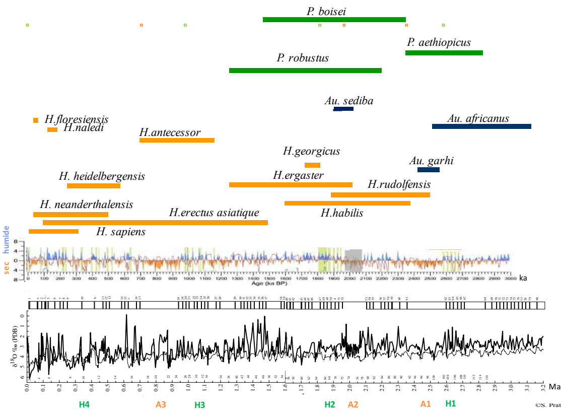
De haut en bas les séries sont: cadre chronologique du genre Homo conçu par Sandrine Prat, série chronologique de l'index humide-sec (bleu-orange) reproduit d'après la figure 8 de (Grant et al. 2017) avec périodes d'augmentation de l'humidité au Sahara et en l'Afrique de l'Est (barres vertes), et séries de l'isotope de l'oxygène et sapropels reproduites d'après la figure 3 de (Kroon et al. 1998).
