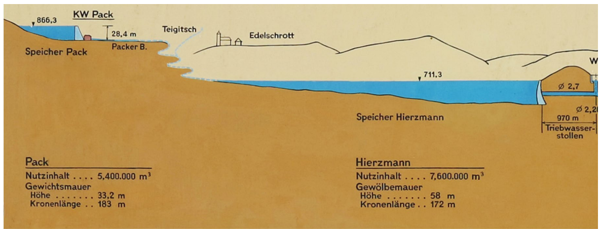
Schematische Darstellung der Teigitschgruppe vom Speicher Pack (links) bis zum Kraftwerk Teigitschmühle (rechts). Clemens Stockner.
