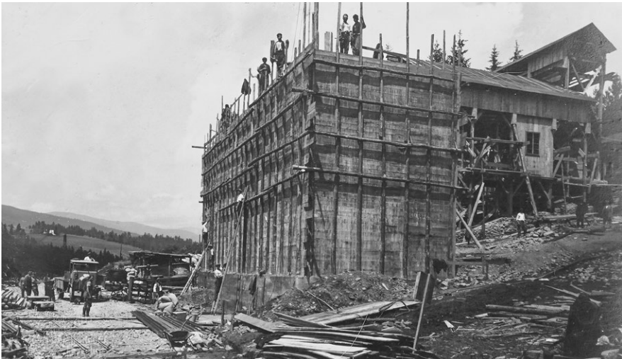
Bauarbeiten bei der Sperre Pack, 1929. Foto Allmann, Graz.
