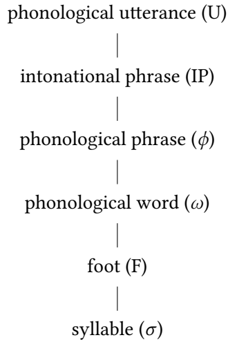
Figure 4.3: Prosodic hierarchy
