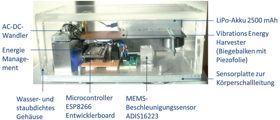
Abb. 4 Bestandteile Sensorknoten [58]
