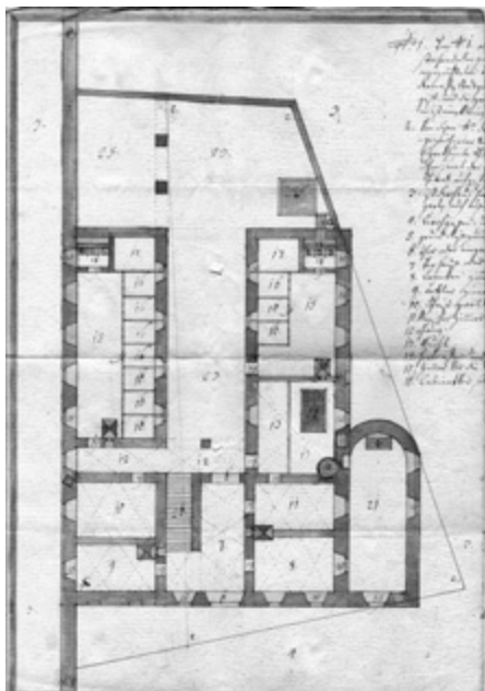
Abb. 84: Bleiburg; „Kumesch“-Plan des Bürgerspitals, Grundriss des Spitals, Teil 1. Die Schlafkammern und die Spitalkirche sind durch Öffnungen miteinander verbunden (Quelle: KLA, Milde Stiftungen I, Sch. 71, Fasz. 931, Nr. 30, undatiert, November 1766).
