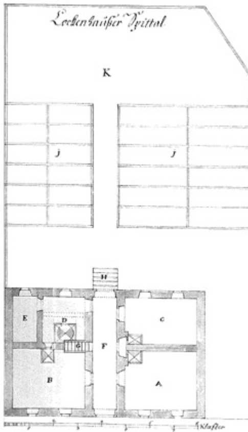
Abb. 142: Lockenhaus; Grundriss des Herrschaftspitals, das sich in unmittelbarer Nähe zur ab 1656 (bis 1669) erbauten Klosterkirche (Augustiner-Eremiten) befindet (BLA, FA Esterházy, Repositorium 82, Fasz. C): Das gebäu ist 8 klaffter lang und 5 klaffter 2 schuh breit, in demselben befinden sich drey zimmer, eine kuchel und eine speis mit einem gang in der mitten, so eine klaffter in der breite hat; der darzu gehörige und anliegende kuchel garten hat 45 klaffter in der länge, auf 9 und 10 klaffter in der breite, wie solches aus dem beygefügtten riß mit mehrern zu ersehen ist: A ist das männerzimmer mit 6 bethern; B das weiberzimmer mit 5 bethern; C ein zimmer mit einem beth, worinnen das spittal weib wohnet, so die kuchel zu besorgen hat; D ist die kuchel; E die speis; F der gang, G die stiegen auf den botend; H die stiegen in den garten; I, J seynd 24 garten bethlen, wovon jeder spittäler 2 geniesset; und H ist ein graß und obst garten, wovon das wenige graß und [I] und obst verkaufft und das geld in zwölf theil zertheilt und einem jeden spittäler ein theil gegeben wird.
