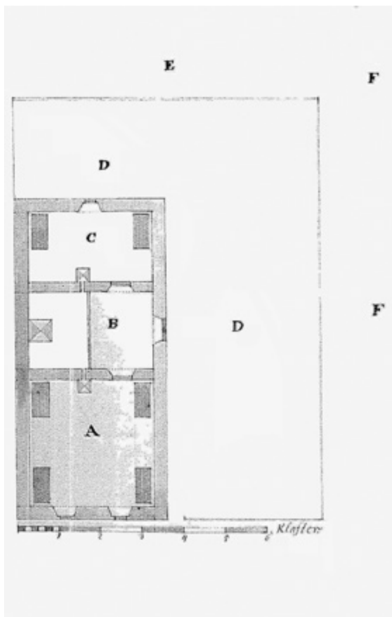
Abb. 144: Pötttsching; Grundriss des Herrschaftspitals, das sich in unmittelbarer Nachbarschaft zur Pfarrkirche befand (BLA, FA Esterházy, Repositorium 82, Fasz. C): Das gebäu bestehet, wie aus dem angefügten riß zu ersehen, aus dem grossen zimmer A mit 4 bethstätten, aus dem kleinern zimmer C mit 2 bethstätten und aus der kuchel B zwischen desn 2 zimmern; dann dem kleinen hoff DD; in FF aber sind 3 halter häusel samt gartl und in E ist des Pötttschinger pfarrers sein garten.
