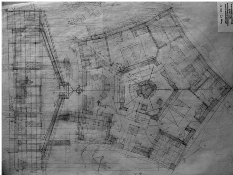
Figura 2.5. Casa Lina. Soluzione iniziale 'h1' su matrice pentagonale. FR, [CD.146/I/SI/H1-1].
