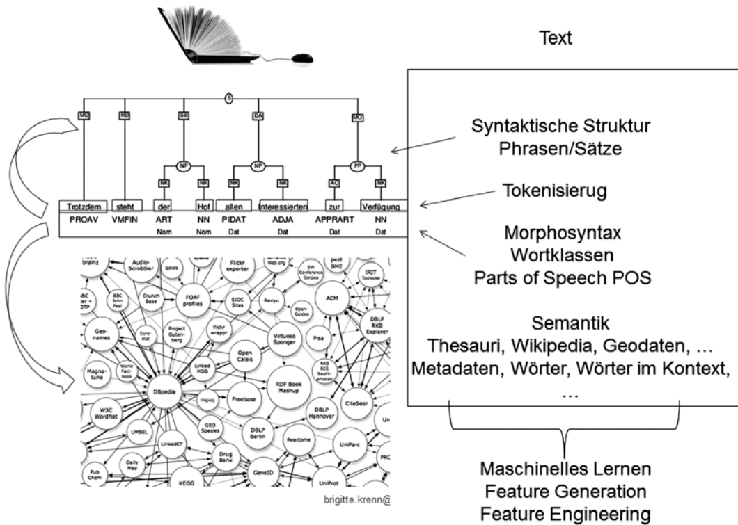
Abb.1: Verarbeitungsstufen in der Textanalyse (Brigitte Krenn).
