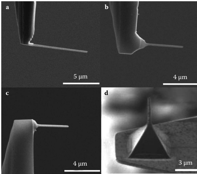
FIGURE 9.14 Actual images of (a) Si, (b) Si-Ti, (c) and (d) tungsten nanoprobes.
