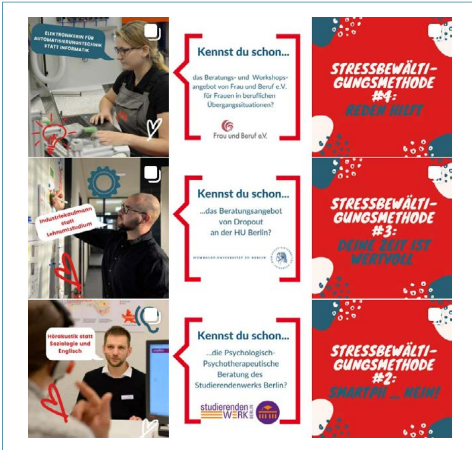
Abbildung 6: Instagram
