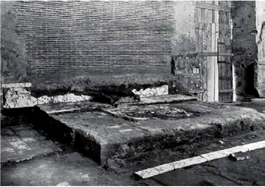
Fig. 90. Detalle del podio de la presidencia de la Curia Iulia .
