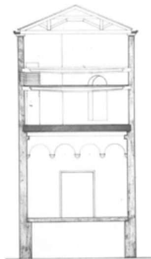
SEZIONE CC
