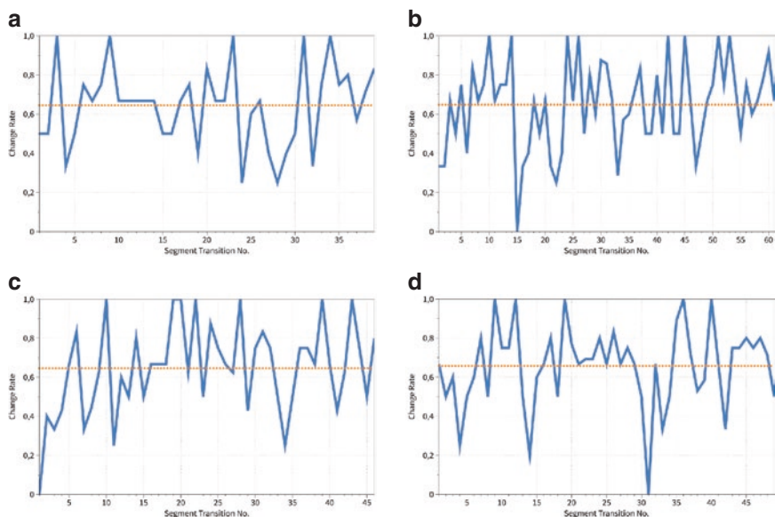
Abb. 20 a. Gottsched: Die Pietisterei (1736) – Mean: 0,64 / SD: 0,20 b. Schiller: Wallensteins Tod (1799) – Mean: 0,65 / SD: 0,22 c. Ganghofer: Der Herrgottschnitzer (1880) – Mean: 0,65 / SD: 0,23 d. Sudermann: Der Bettler von Syrakus (1911) – Mean: 0,66 / SD: 0,21
