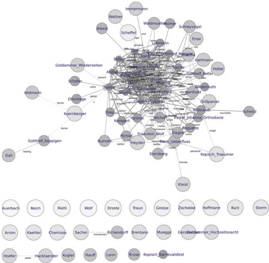
Abb. 9 Gleiches Netzwerk wie Abb. 6, 7 und 8. Dargestellt werden die Wörter, die beide Texte am stärksten unterscheiden 31
