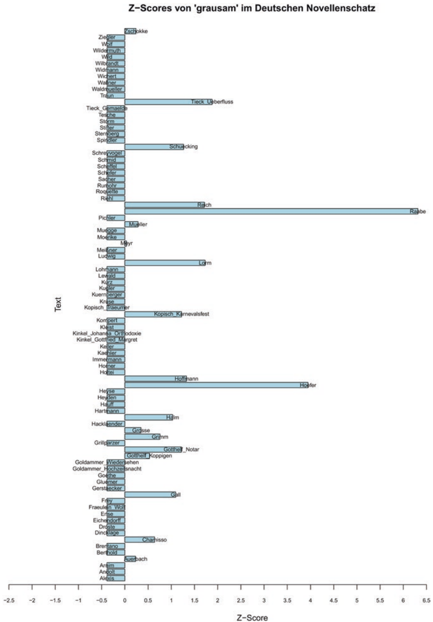
Abb. 10 Z-Score-Profil für „grausam“ 33
