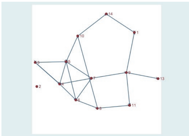
Abbildung 3: Netzwerkplot
