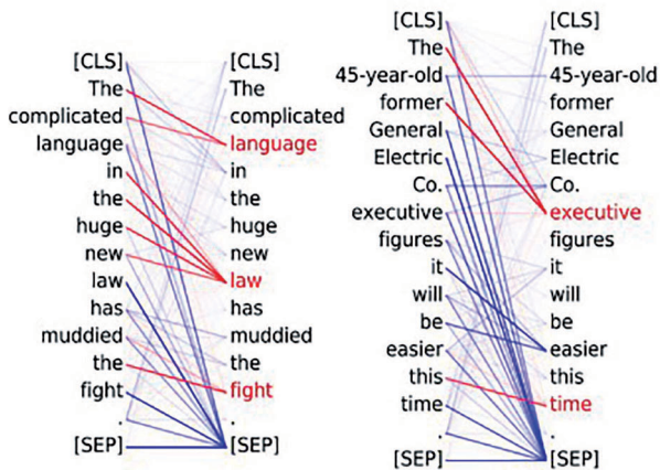
Abbildung 2: Beispiel für die Aufmerksamkeit eines Attention Heads. 46
