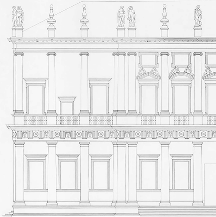
C.I.S.A. A. PALLADIO VICENZA PALAZZO CHERICATI PROSPETTO SULLA PIAZZA SCALA 1:50 DES. 30-15 GIUG. 68
