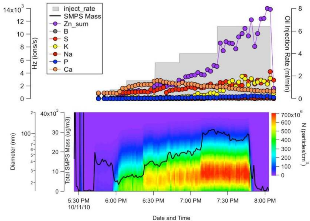
Abbildung 2.14: Öleindosierung, Aschebelastung und Partikelgrößenverteilung in einem Grundlagenversuch bei einem mit Diesel betriebenen Verbrenner [189]
