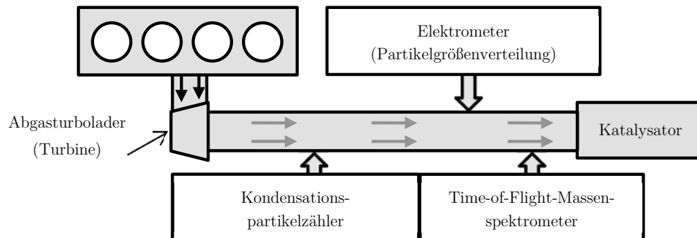
Abbildung 4.1: Schematische Darstellung der Messpositionen im Rohabgas
