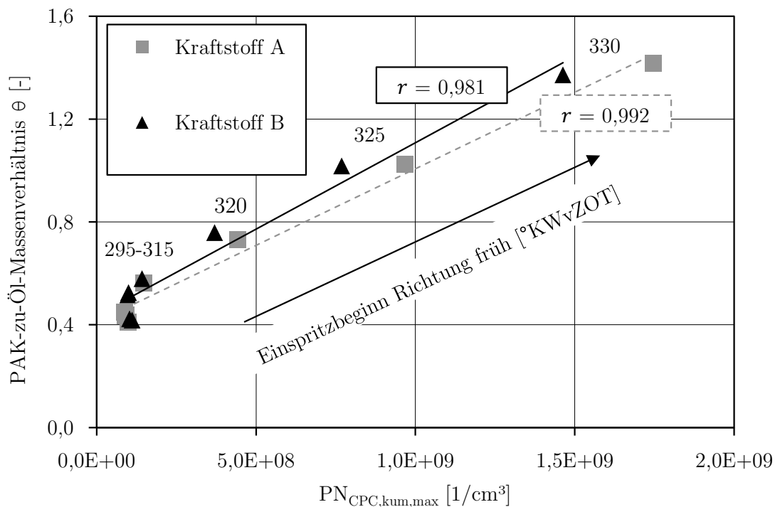
Abbildung 5.11: Korrelationen der PAK-zu-Öl-Massenverhältnisse und der Partikelanzahl der beiden Kraftstoffe A und B mit Öl B im stationären Motorbetrieb bei 2000 min -1 , 90 Nm mit Variation des Einspritzbeginns (ESB, 295 - 330 °KWvZOT)
