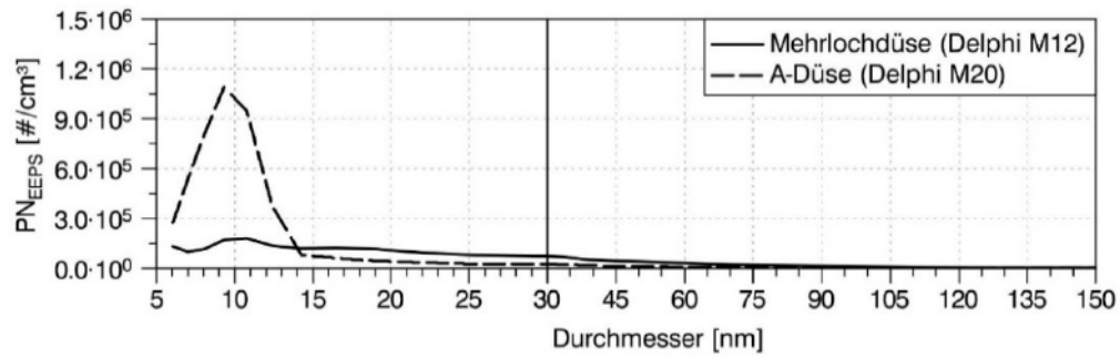
Abbildung 2.13: Partikelgrößenverteilung für Mehrloch- und A-Düse im Katalysatorheizen [44]
