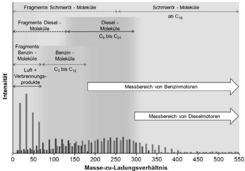
Abbildung 3.3: Massenspektrum und Messbereiche für Otto- und Dieselmotoren [106]
