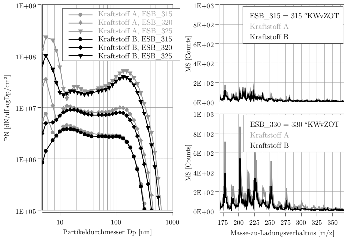
Abbildung 4.17: Kraftstoffvergleich für Kraftstoff A und B bezüglich Partikelgrößenverteilung und Massenspektrum bei unterschiedlichem Einspritzbeginn bei \lambda = 1 und 72 °C Kühlwassertemperatur im Stationärpunkt 2000 \text{ min}^{-1} , 90 \text{ Nm}
