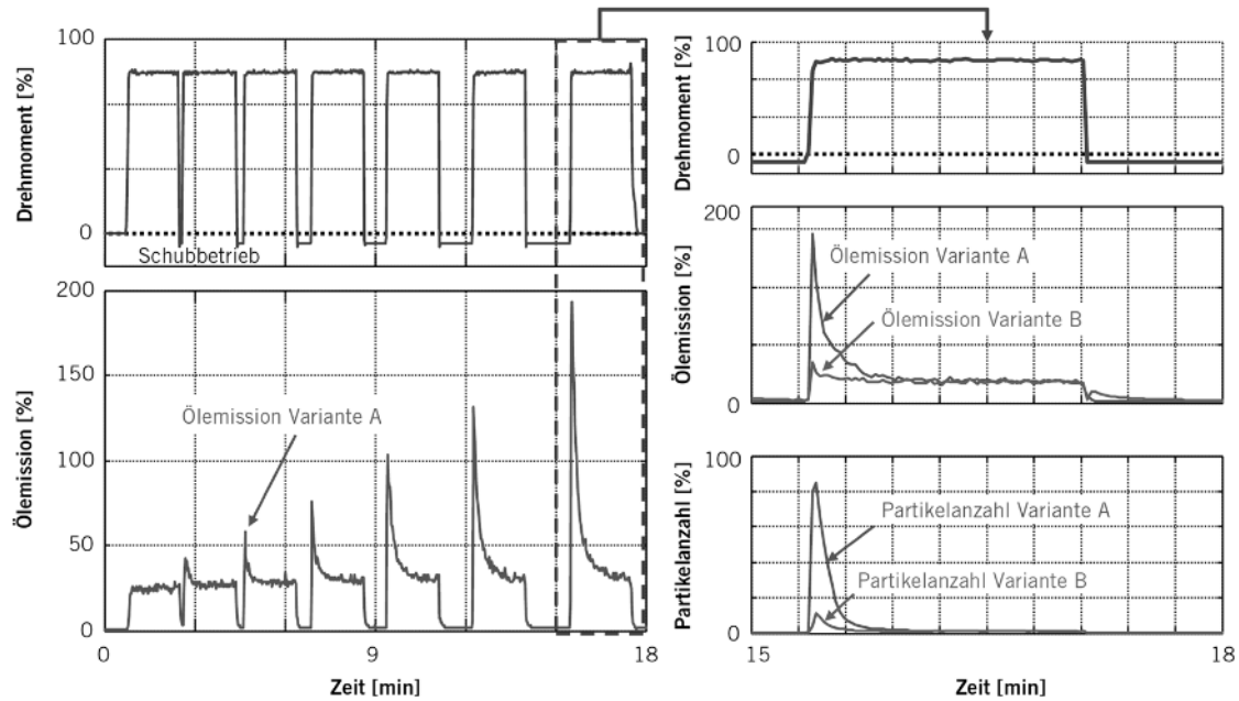
Abbildung 4.6: Öl- und Partikelemissionen bei Schub-Last-Wechseln für zwei Hardwarevarianten [187]
