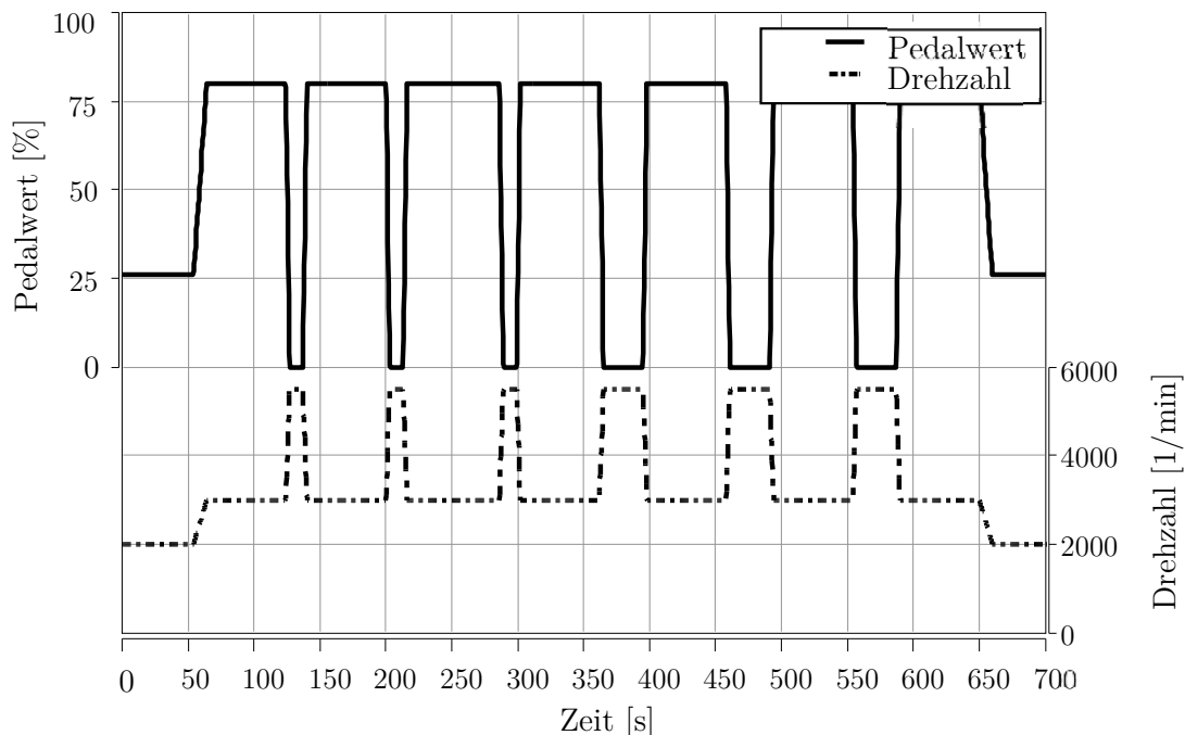
Abbildung 4.4: Betriebsprofil des synthetischen Dynamikzyklus mit Schub-Last-Wechsel
