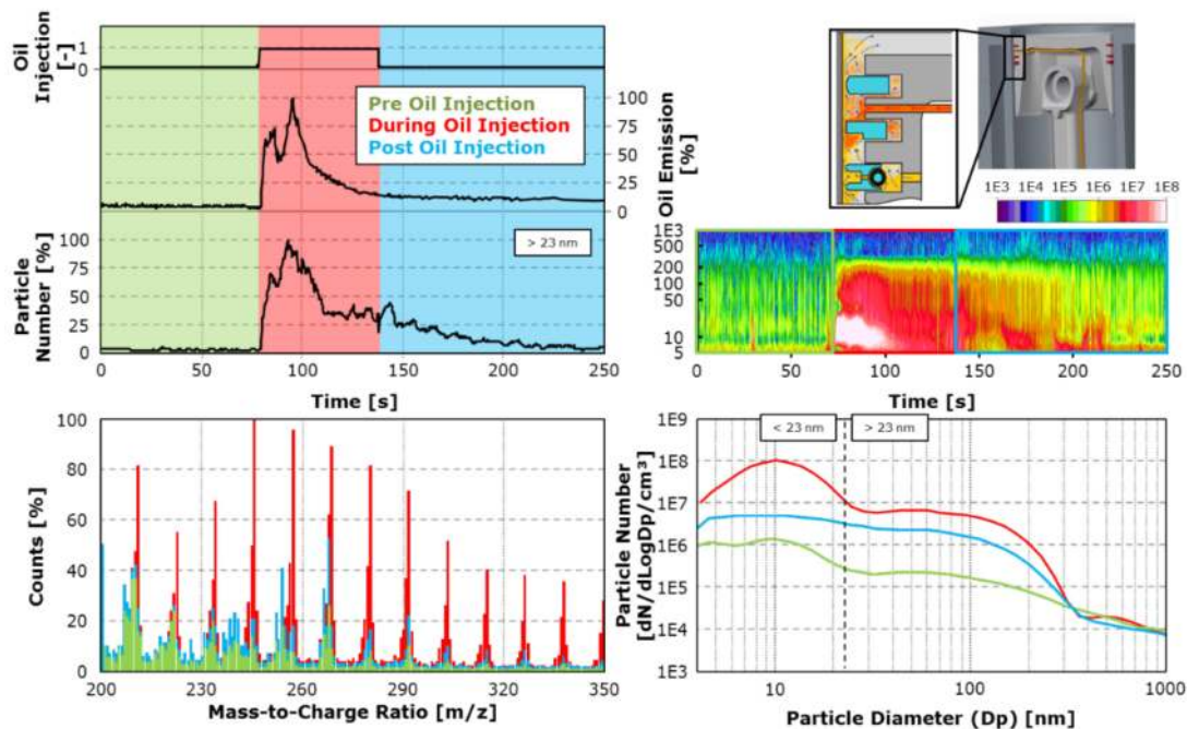
Abbildung 2.11: Emissionseinfluss der Öleindosierung im Zwischenringbereich [185]
