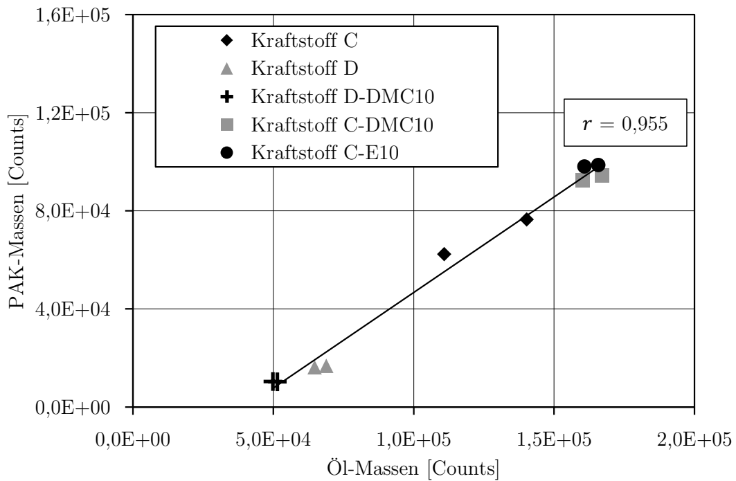
Abbildung 5.6: Korrelation der Öl- und PAK-Massen (Öl B; Kraftstoffe C, C-E10, C-DMC10, D und D-DMC10) im hochdynamischen RDE-Ausschnitt (nur Lastphase 2)
