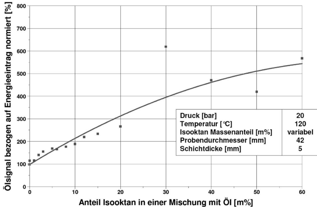
Abbildung 2.7: Kraftstoffeinfluss auf die Ölverdampfung bei 120°C [137]
