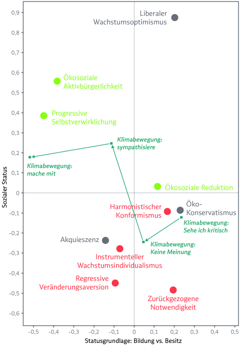
Abbildung 22: Haltung zu und Aktivität in der Klimabewegung, Verteilung der Mittelpunkte der Antwortoptionen im Raum
