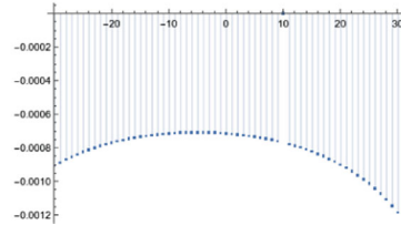
(d) Summands in (16.2.7) for (\lambda_i, \lambda_j) = (10, 0)
