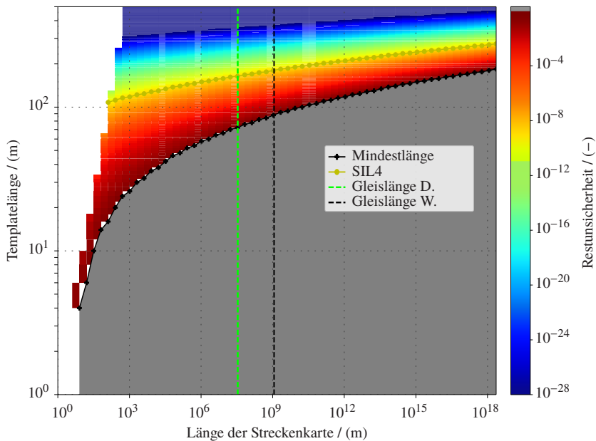
Abbildung 5.3: Templatelänge, die für eine eindeutige Positionsbestimmung erforderlich ist. Die vertikalen Linien entsprechen der gesamten deutschen (grün; ca. 61000 km) und weltweiten (schwarz; ca. 1148186 km) Gleisstreckenlänge [73], [74].
