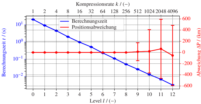
Abbildung 5.4: Berechnungszeit und Abweichung zur Referenzposition in Abhängigkeit der dazugehörigen Wavelet-Koeffizienten für das jeweilige Level l . Auf einer Streckenkarte von 1342 km wurden für jeweils 100 unterschiedliche Templates (mit einer Länge von jeweils 200 m) die Positionen ermittelt.
