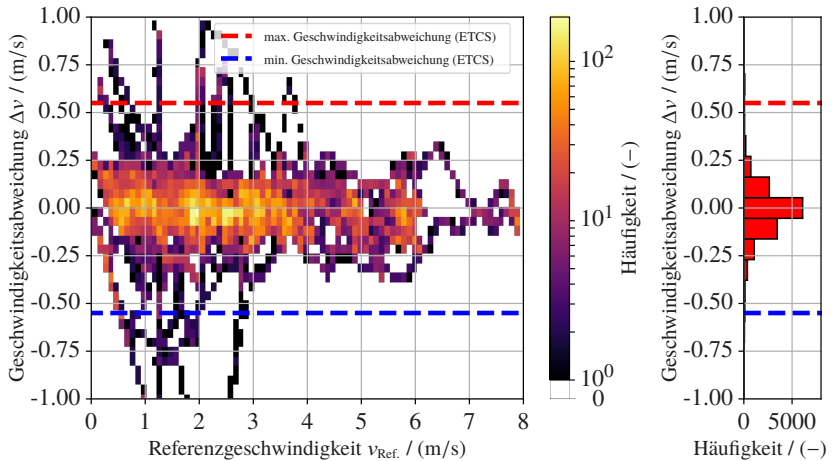
Abbildung 3.13: Links: Häufigkeit der Geschwindigkeitsabweichung aufgetragen über die Referenzgeschwindigkeit v_{Ref} des Schienenfahrzeugs für die Streckenabschnitte ID = 1 bis 33. Rechts: Histogramm der Häufigkeit akkumuliert über alle Geschwindigkeiten. Die blau und rot gestrichelte Linie kennzeichnen die minimale und maximale zulässige Geschwindigkeitsabweichung nach ETCS [7].
