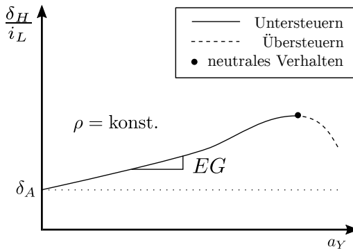
Abbildung 2.2: Eigenlenkverhalten – Lenkgradwinkel über Querbeschleunigung ([119], nach Heiöing et al. [36], Mitschke und Wallentowitz [68])
