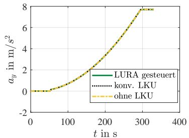
(d) Querbeschleunigung a_y .
