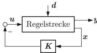
Abbildung 2.12: Regelung mit Zustandsrückführung. [63]
