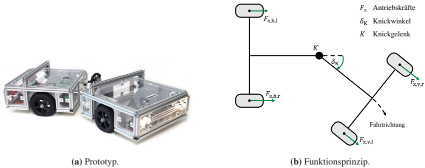
Abbildung 7.4: Prototyp und Funktionsprinzip eines Knicklenkers mit Nutzung radselektiver Antriebe zur Lenkung.
