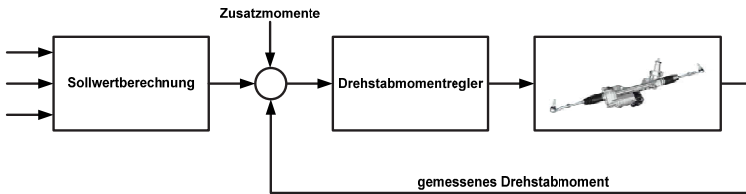
Abbildung 3.3: Regelkreis bei modernen EPS Regelungskonzepten, die auf der Regelung des Fahrermoments basieren. [75]
