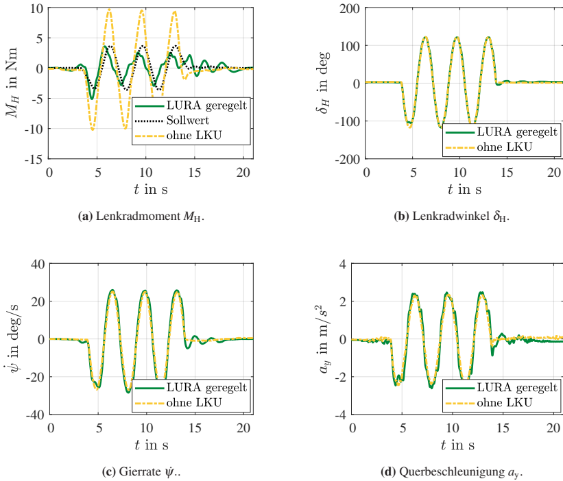
Abbildung 6.4: Validierungsergebnisse des Dauersinus ( f = 0,3\text{Hz} ) mit geregelter LURA.
