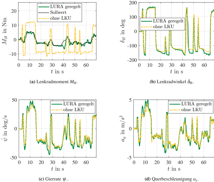
Abbildung 6.9: Repräsentativer Ausschnitt der Validierungsergebnisse bei einer Realfahrt mit geregelter LURA.
