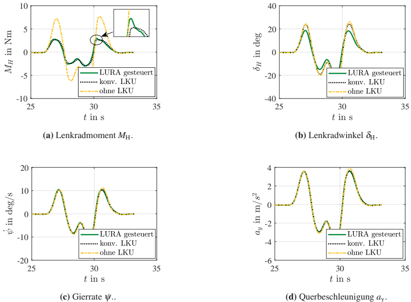
Abbildung 5.11: Simulationsergebnisse des doppelten Spurwechsels mit gesteuerter LURA.
