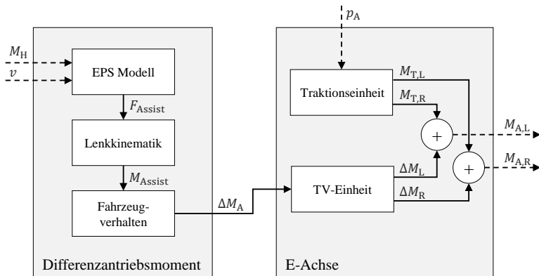
Abbildung 7.2: Strukturbild zur Steuerung der Lenkkraftunterstützung mittels elektrischer Achse.
