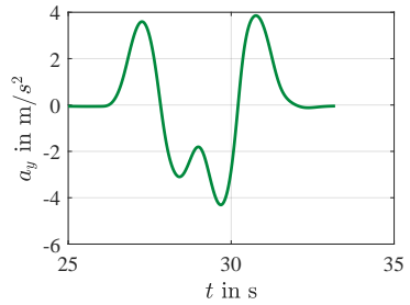
(b) Querbeschleunigung a_y .
