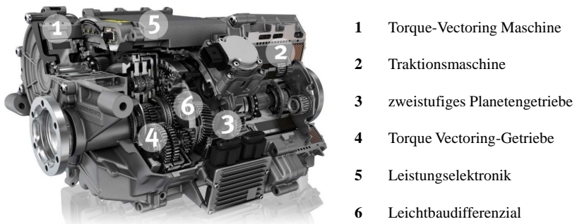
Abbildung 7.1: Elektrische Achse (aus [82], bearb.).
