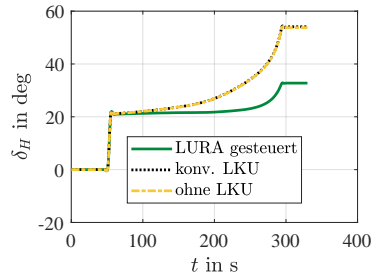
(b) Lenkradwinkel \delta_H .
