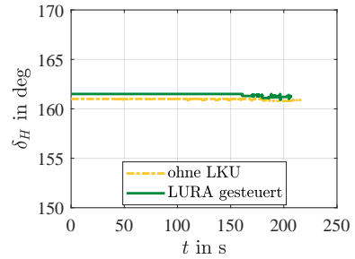
(b) Lenkradwinkel \delta_H .
