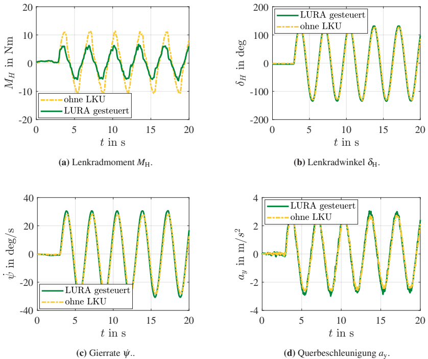
Abbildung 6.3: Validierungsergebnisse des Dauersinus ( f = 0,3\text{Hz} ) mit gesteuerter LURA.
