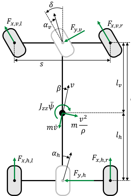
Abbildung 4.5: Erweitertes Fahrzeugmodell zur Abbildung radselektiver Antriebskräfte.
