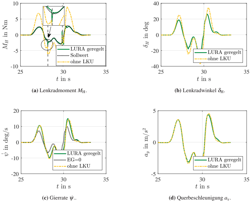
Abbildung 5.17: Simulationsergebnisse bei Lenkung auf \mu -Split mit geregelter LURA.
