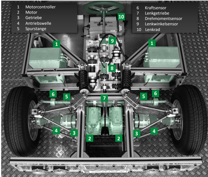
Abbildung 4.3: Lenk- und Antriebssystem des Demonstratorfahrzeugs ELF++.
