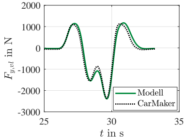
(a) Seitenkraft F_{y,vl} vorne links.
