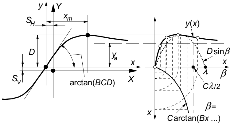
Abbildung 4.7: Magic Formula [73].
