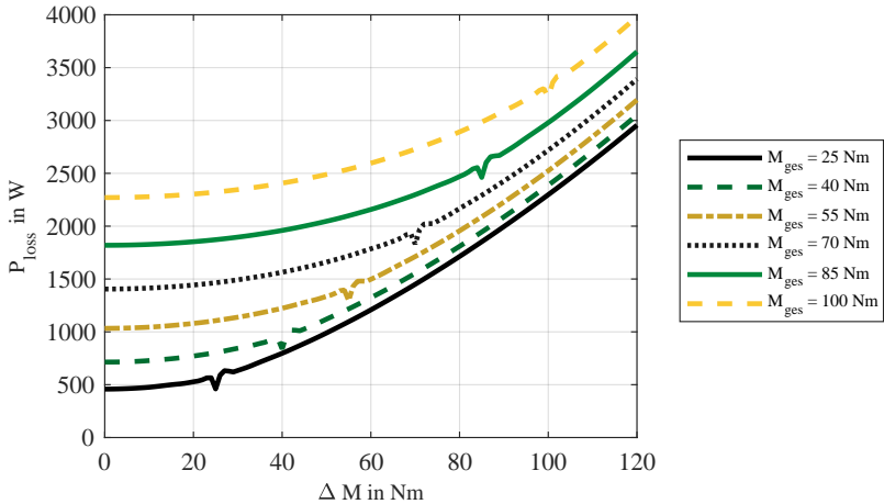
Abbildung 4.13: Gesamtverluste der E-Maschinen in Abhängigkeit des Differenzmoments.
