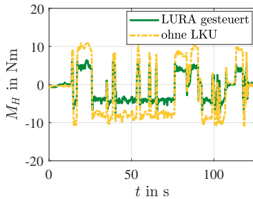
(a) Lenkradmoment M_H .
