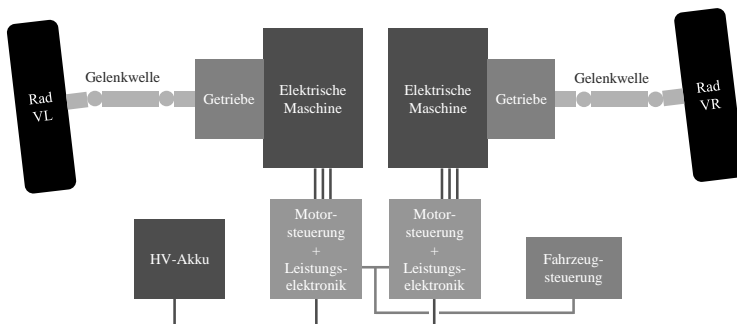
Abbildung 5.1: Schematische Darstellung des Antriebsstrangs im Simulationsmodell.
