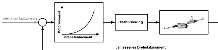
Abbildung 3.2: Regelkreis bei klassischem EPS Regelungskonzept. [75]
