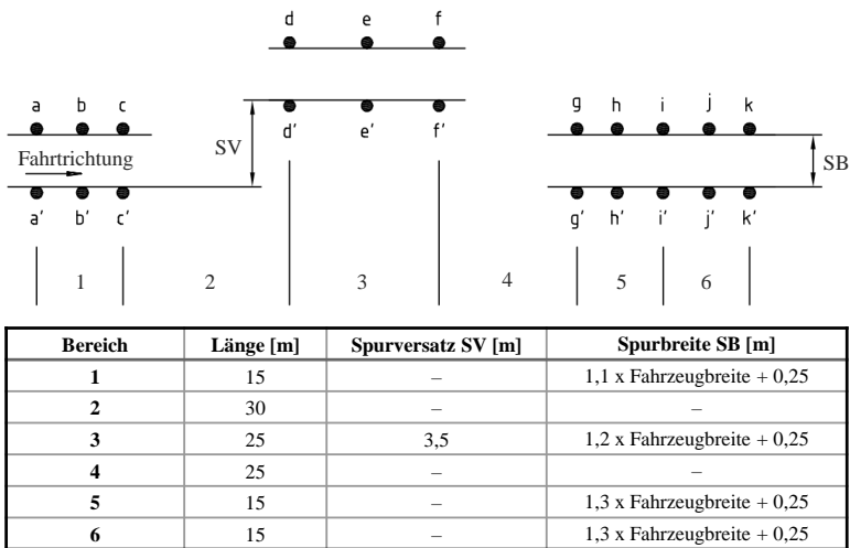
Abbildung 5.10: Streckenaufbau doppelter Spurwechsel (nach [43]).
