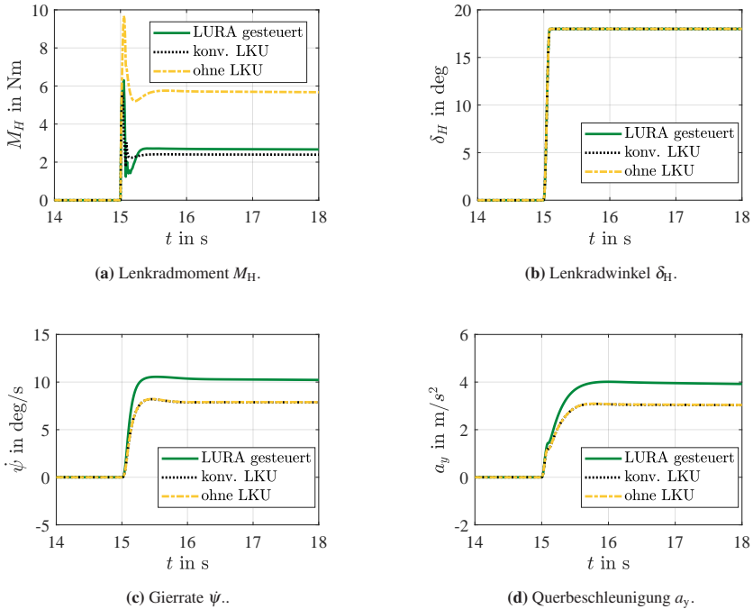
Abbildung 5.13: Simulationsergebnisse des Lenkwinkelsprungs nach ISO 7401 mit gesteuerter LURA.
