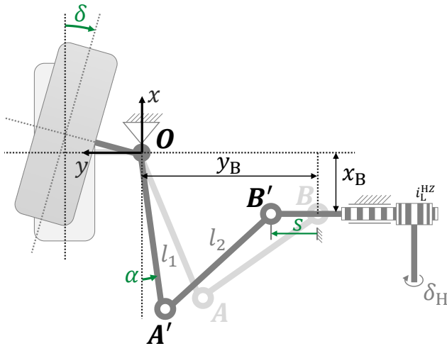
Abbildung 4.8: Zusammenhänge zwischen Zahnstangen- und Lenkbewegung am linken Vorderrad.
