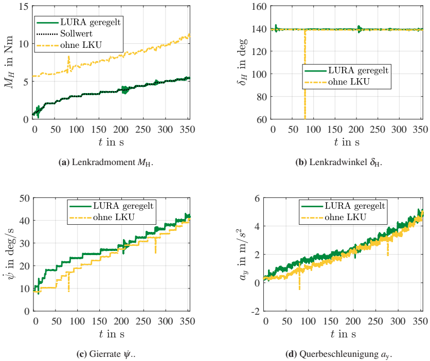
Abbildung 6.2: Validierungsergebnisse der stationären Kreisfahrt mit geregelter LURA.
