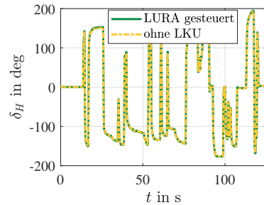
(b) Lenkradwinkel \delta_H .
