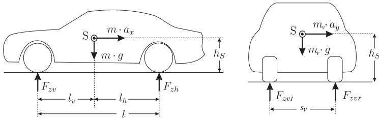
Abbildung 4.6: Vertikalkräfte in Seitenansicht (links) und Rückansicht auf vordere Fahrzeughälfte (rechts) (aus [137], nach von Vietinghoff [98]).
