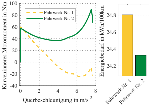
Abbildung 5.25: Motormoment des kurveninneren Antriebs und Energiebedarfsreduktion ( \Delta E gemäß Abschnitt 5.7) durch Nutzung eines Fahrwerks mit größerem Störkrafthebelarm (nach [112]).
