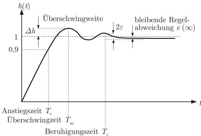
Abbildung 2.13: Führungsübergangsfunktion des Regelkreises mit Kennzeichnung wichtiger Kennwerte. [62]
