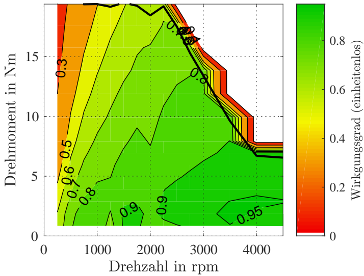
Abbildung A.2: Wirkungsgradkennfeld der elektrischen Antriebe inkl. Leistungselektronik des Demonstratorfahrzeugs ELF++.
