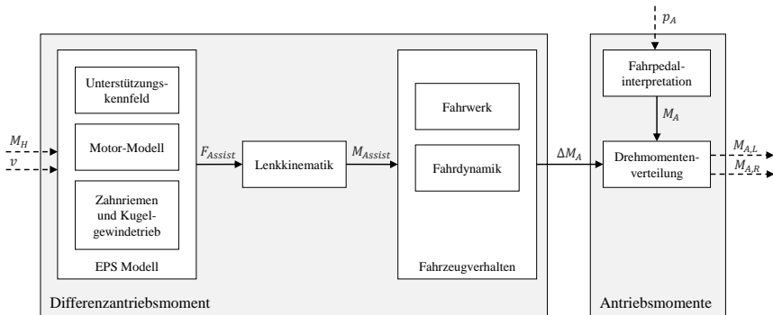
Abbildung 4.9: Open-Loop Steuerung der Lenkkraftunterstützung mittels radselektiver Antriebe.
