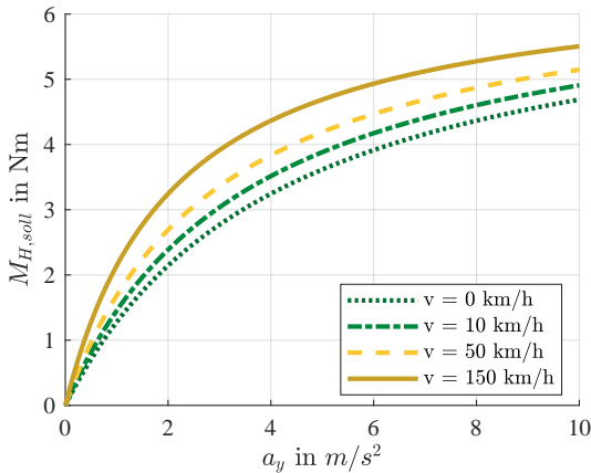
Abbildung 4.12: Soll-Lenkradmoment in Abhängigkeit der Fahrzeuggeschwindigkeit.
