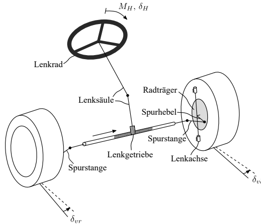
Abbildung 2.4: Schematischer Aufbau einer Lenkung (nach [20] aus [119], bearb.).
