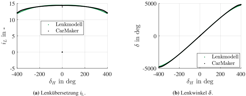
Abbildung A.9: Lenkübersetzung und Lenkwinkel über Lenkradwinkel \delta_H .
