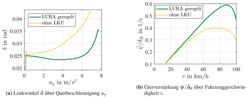
Abbildung 5.5: Simulationsergebnisse der stationären Kreisfahrt mit geregelter LURA.
