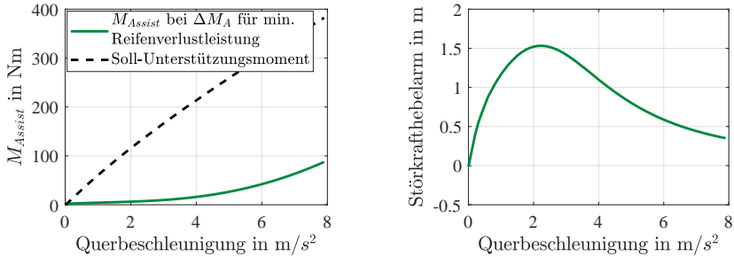
(a) Unterstützungsmoment bei Differenzmoment mit Ziel minimaler Reifenverluste.
