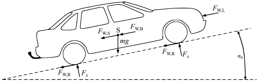
Abbildung 2.3: Fahrwiderstände bei beschleunigter Fahrt und Steigung (nach Gauterin und Unrau [30]).
