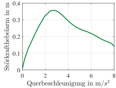
(b) Störkrafthebelarm über Querbeschleunigung für EG = 0 .
