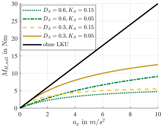
Abbildung 4.11: Einflüsse von Gradientenfaktor D_A und Degressivitätsfaktor K_A auf das Soll-Lenkradmoment.
