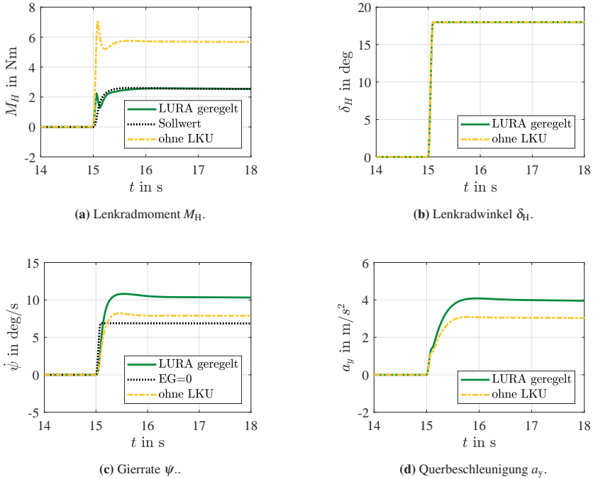
Abbildung 5.14: Simulationsergebnisse des Lenkwinkelsprungs nach ISO 7401 mit geregelter LURA.
