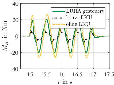
(a) Lenkradmoment M_H bei f_\delta = 2 Hz.
