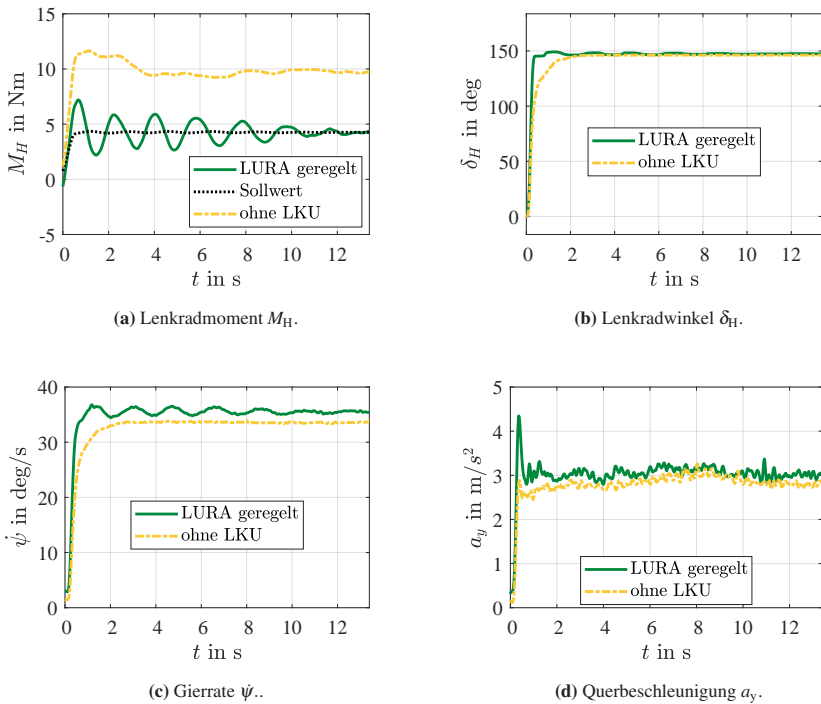
Abbildung 6.6: Validierungsergebnisse des Lenkwinkelsprungs nach ISO 7401 mit geregelter LURA.
