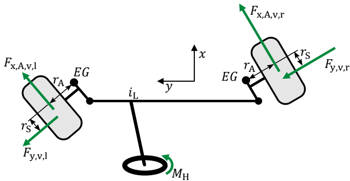
Abbildung 2.10: Funktionsprinzip einer Lenkkräftunterstützung mittels radselektiver Antriebe.
