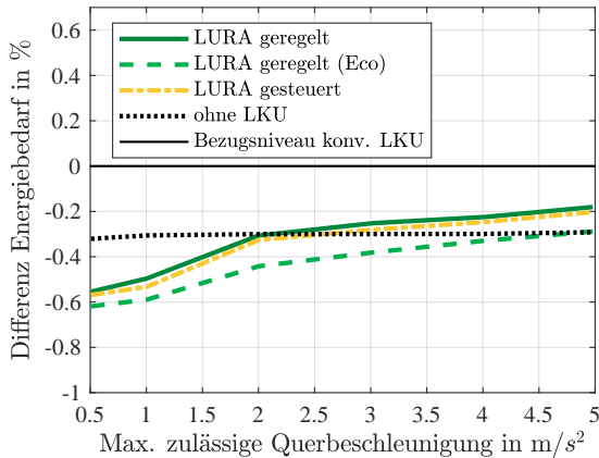
Abbildung 5.21: Differenz des Energiebedarfs im Bezug zur Nutzung einer konventionellen LKU in Abhängigkeit der maximal zulässigen Querbeschleunigung.
