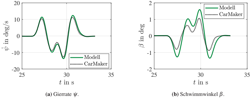
Abbildung A.8: Validierung von Gierrate und Schwimmwinkel beim doppelten Spurwechsel.
