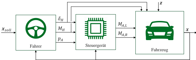
Abbildung 4.1: Regelungssystem Fahrer und Fahrzeug mit radselektiven Antrieben an der Vorderachse.
