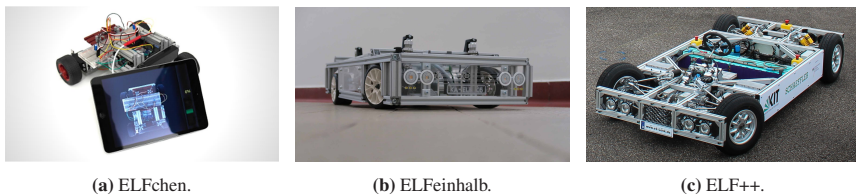
Abbildung 4.2: Demonstratorfahrzeuge zur Entwicklung von Lenkungs- und Fahrwerkskonzepten.
