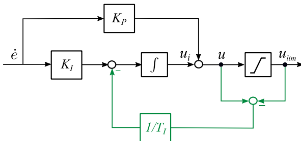
Abbildung 4.18: PI-Regler mit Anti-Windup Maßnahme (aus [137] nach Horn [40]).
