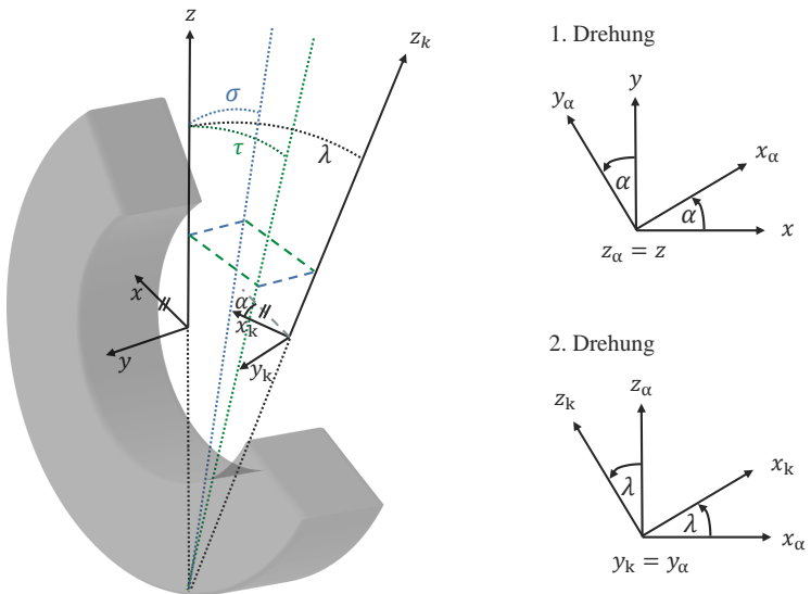
Abbildung A.1: Räumliche Darstellung der Lenkachse.
