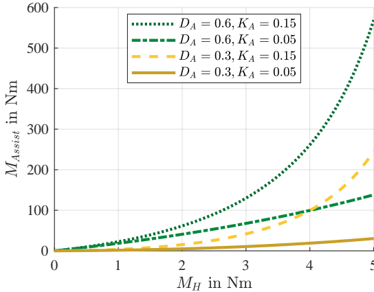
Abbildung 4.10: Einflüsse von Gradientenfaktor D_A und Degressivitätsfaktor K_A auf das Unterstützungsmoment.
