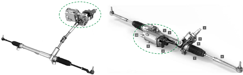
Abbildung 2.9: Lenksäulenbasiertes (links) und achsparalleles (rechts) elektromechanisches Lenkkraftunterstützungssystem (Quelle: Springer2014 [95] und Bosch2015 [81]).
