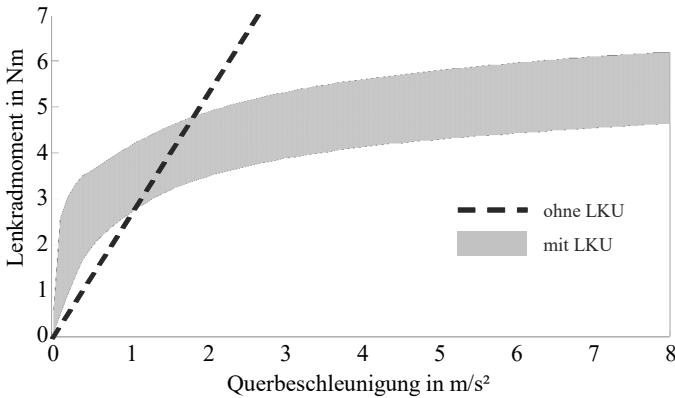
Abbildung 2.8: Lenkradmoment in Abhängigkeit der Querbesehleunigung (nach Pfeffer und Harrer [76]).
