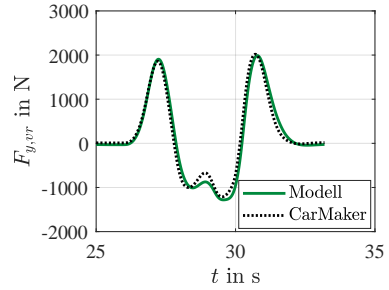
(b) Seitenkraft F_{y,vr} vorne rechts.
