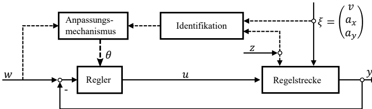
Abbildung 4.16: Gesteuerte Adaption (nach [123, 96]).
