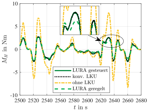
Abbildung 5.22: Repräsentativer Ausschnitt der Simulationsergebnisse bei einer RDE Fahrt mit geregelter und gesteuerter LURA im Vergleich.
