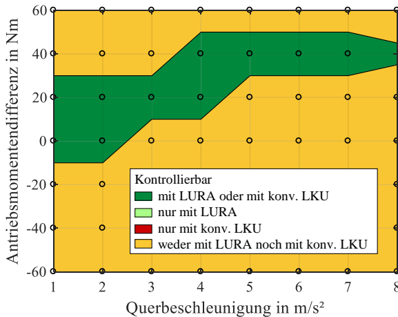
Abbildung 5.24: Vergleich der Fehlertoleranz von LURA und konv. LKU ([129], bearb.).
