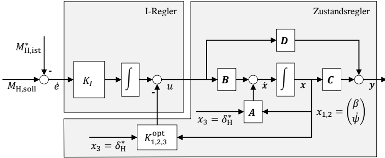
Abbildung 4.15: Ausgangsstruktur der Regelung.
