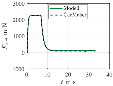
(a) Längskraft F_{x,vl} vorne links.
