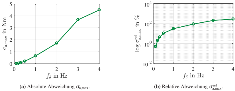
Abbildung 5.9: Abweichung des geregelt en Lenkradmoments vom Soll-Moment in Abhängigkeit der Lenkfrequenz.
