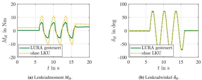
Abbildung 6.7: Validierungsergebnisse bei Lenken mit Dauersinus ( f = 0,3 \text{ Hz} ) im Stand bei gesteuerter LURA.
