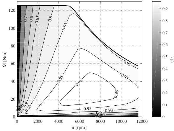
Abbildung A.3: Wirkungsgradkennfeld der elektrischen Antriebe.
