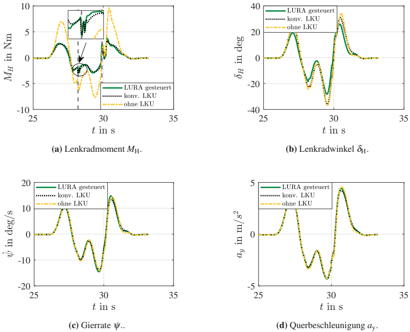
Abbildung 5.16: Simulationsergebnisse bei Lenkung auf \mu -Split mit gesteuerter LURA.
