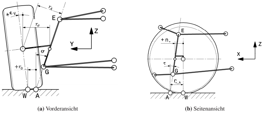
Abbildung 2.5: Kenngößen von Lenkgeometrien am Beispiel eines Doppeldreiecklenkers (Matschinsky [65], bearb.).
