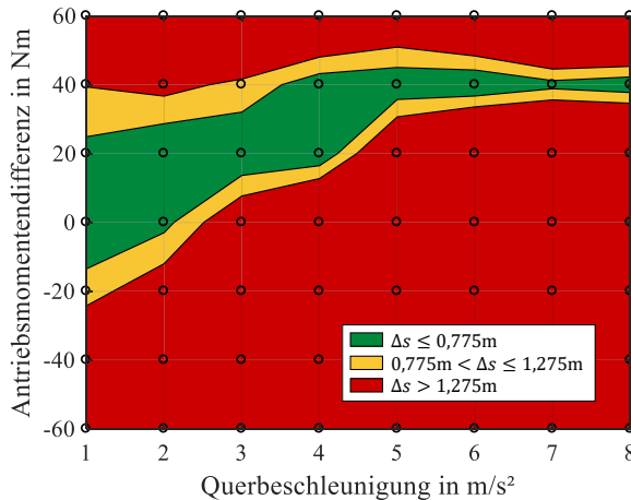
Abbildung 5.23: Absolute Abweichung von der Soll-Fahrspur aufgrund eines plötzlichen Sprungs des Antriebsdifferenzmoments der Lenkkraftunterstützung mittels radselektiver Antriebe ([129], bearb.).
