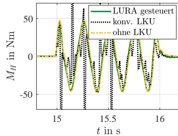
(b) Lenkradmoment M_H bei f_\delta = 4 Hz.
