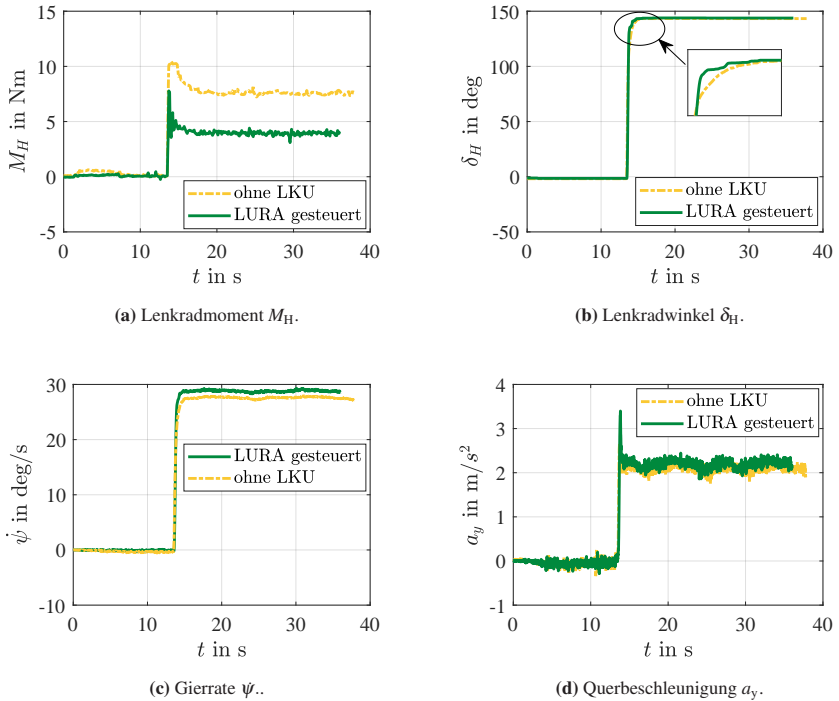
Abbildung 6.5: Validierungsergebnisse des Lenkwinkelsprungs nach ISO 7401 mit gesteuerter LURA.
