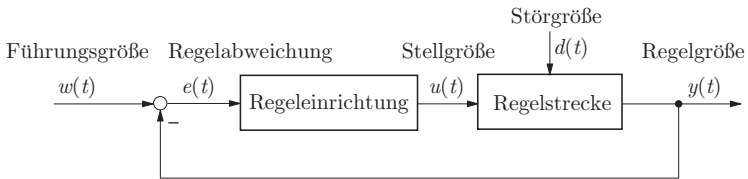
Abbildung 2.11: Grundstruktur eines Regelkreises. [62]
