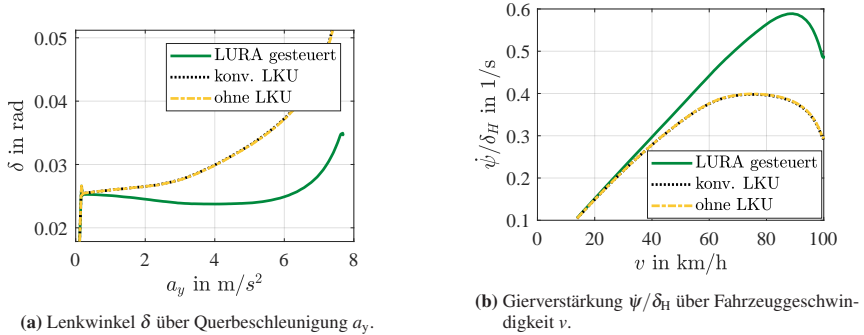
Abbildung 5.3: Simulationsergebnisse der stationären Kreisfahrt mit gesteuerter LURA.
