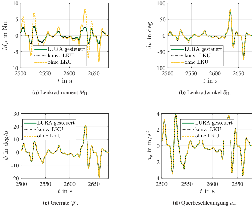
Abbildung 5.19: Repräsentativer Ausschnitt der Simulationsergebnisse einer RDE Fahrt mit gesteuerter LURA.
