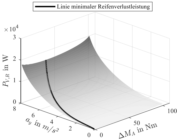
Abbildung 4.14: Reifenverlustleistung über Differenzantriebsmoment und Querbeschleunigungen bei einer quasi-stationären Kreisfahrt.
