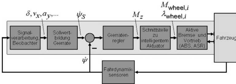
Abbildung 3.1: Regelungstechnisches Strukturbild der ESP-Querdyamikregelung. [50]
