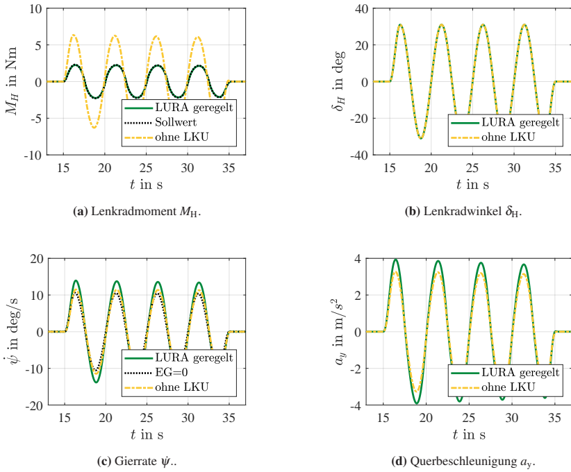
Abbildung 5.8: Simulationsergebnisse des Dauersinus ( f_\delta = 0,2\text{Hz} ) mit geregelter LURA.
