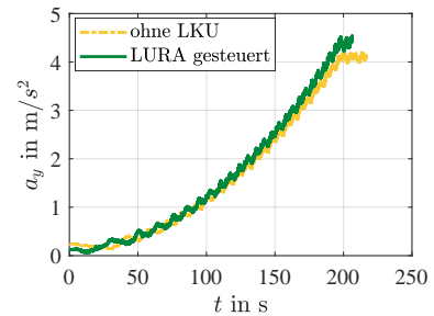
(d) Querbeschleunigung a_y .
