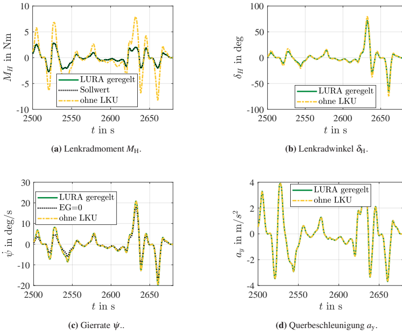
Abbildung 5.20: Repräsentativer Ausschnitt der Simulationsergebnisse einer RDE Fahrt mit geregelter LURA.
