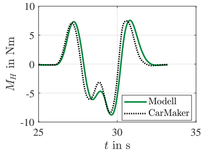
Abbildung A.10: Verlauf des Lenkradmoments M_H beim doppelten Spurwechsel.
