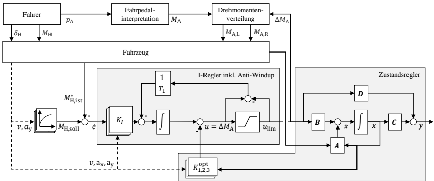
Abbildung 4.19: Vollständige Regelungsstruktur.
