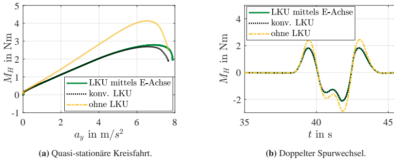
Abbildung 7.3: Vergleich der Lenkradmomente M_H bei Nutzung einer konventionellen LKU und Nutzung der Lenkkraftunterstützung mittels E-Achse.
