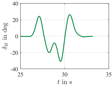
(a) Lenkradwinkel \delta_H .
