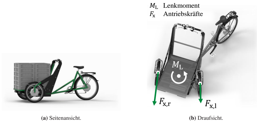
Abbildung 7.5: Designvorschlag eines dreirädrigen Lastenrads mit Nutzung radselektiver Radnabenantriebe zur Lenkung/Lenkkräfteunterstützung. [78]
