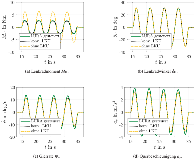
Abbildung 5.6: Simulationsergebnisse des Dauersinus ( f_{\delta} = 0,2\text{Hz} ) mit gesteuerter LURA.
