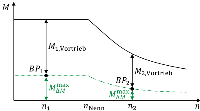
Abbildung 4.17: Stellgrößen in Abhängigkeit des aktuellen Betriebspunkts.
