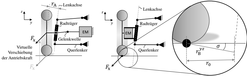
Abbildung 2.7: Wirksame Hebelarme bei innen liegendem (links) und außen liegendem Antrieb (rechts). Projektion in y-z-Ebene.
