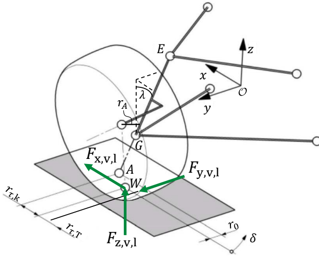
Abbildung 2.6: Kräfte am linken Vorderrad (nach Pfeffer und Harrer [75], basierend auf Matschinsky [65]).
