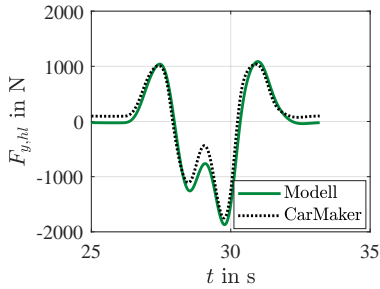
(c) Seitenkraft F_{y,hl} hinten links.
