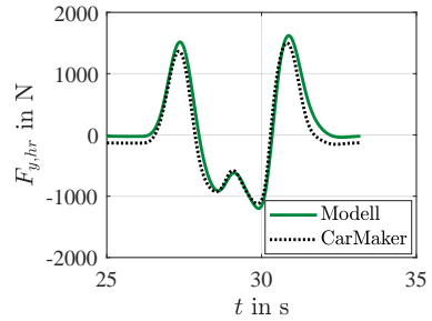
(d) Seitenkraft F_{y,hr} vorne rechts.
