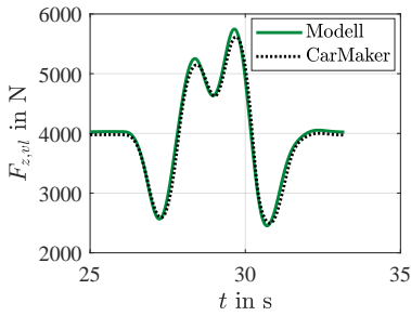
(a) Radlast F_{z,vl} vorne links.
