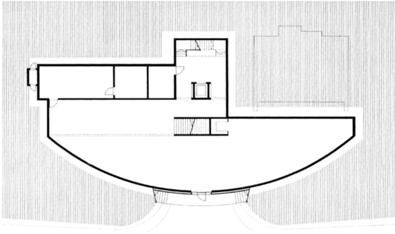
Abb. 5: Mario Botta: Grundriss des Centre Dürrenmatt. Unterstes Geschoss mit dem großen Ausstellungsraum, 1998)
