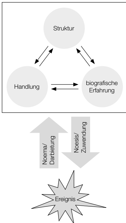
Abb. 3: Detaillierte Darstellung von Gegenwartsmoment 1: Verhältnis von Ereignis und Erleben unter Berücksichtigung von Noema und Noesis
