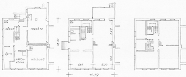
Abb. 148. Keller-, Erd- und Obergeschößgrundriß des Kopfbaues der gleichen Hausreihe
