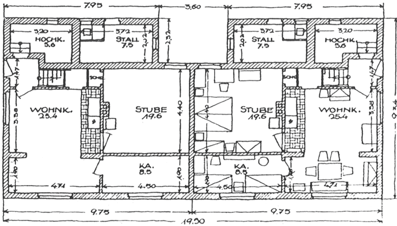
Abb. 12: Erdgeschossegrundriß des Doppelhauses Gr. II, Form 14 L , Bl. 1 : 200.
