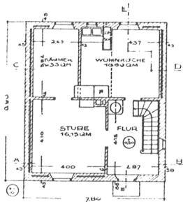
Abb. 1 Erdgeschoßgrundriß des Types Gruppe I, Typ 1, Maßstab 1:200.
