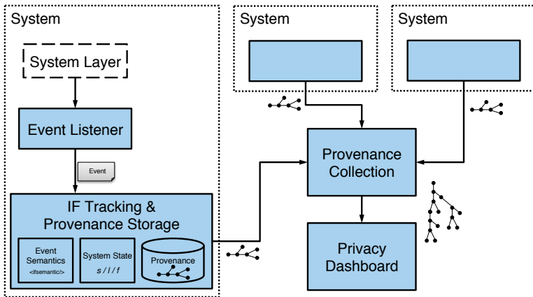
Abbildung 8.7: Aggregation verteilter Personal-Data-Provenance
