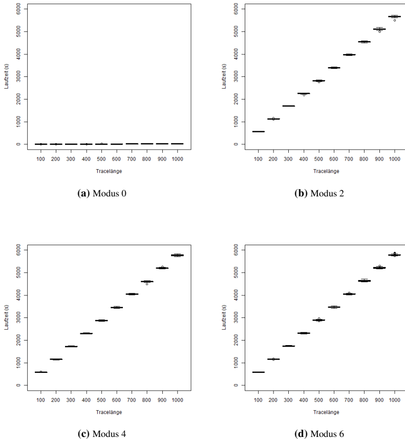
Abbildung 7.2: Laufzeit in Abhängigkeit von der Tracelänge (10 personenbezogene Daten, 100 KB Dateien)
