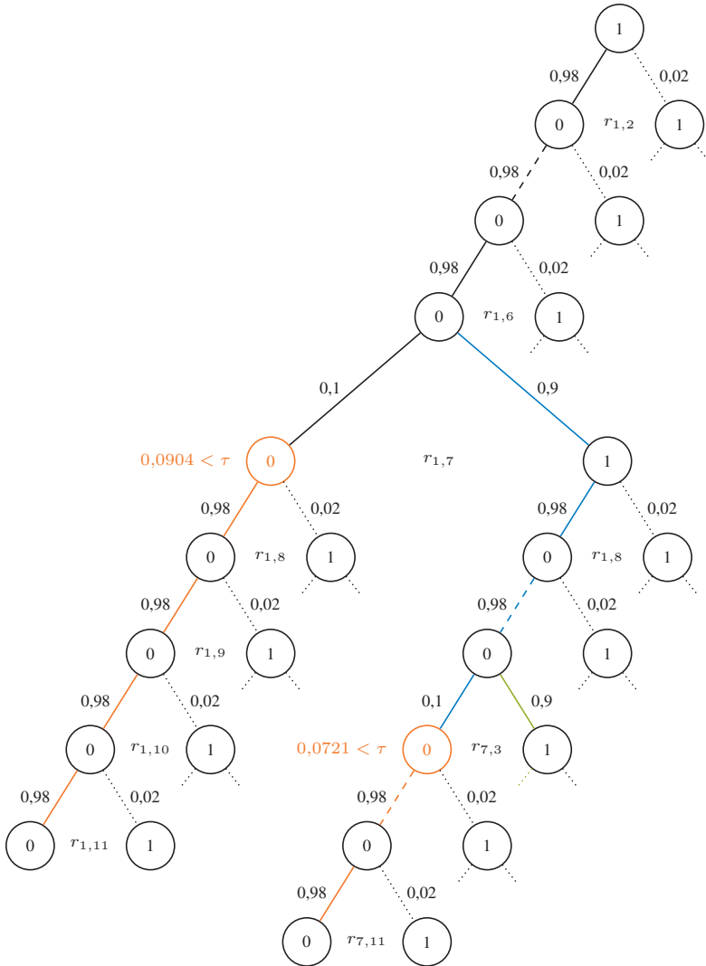
Abbildung 9.4: Wahrscheinlichkeitsbaum für \theta_{14} , ausgehend von c_1 , mit angedeuteter Tiefensuche (erste, zweite und dritte Iteration sowie die Suche nach dem jeweiligen Repräsentanten) für \tau = 0,1
