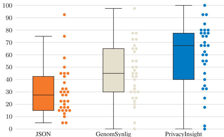
Abbildung 12.3: SUS-Score der drei Vergleichsverfahren
