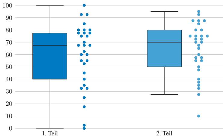
Abbildung 12.4: SUS-Score von PrivacyInsight im ersten und zweiten Teil
