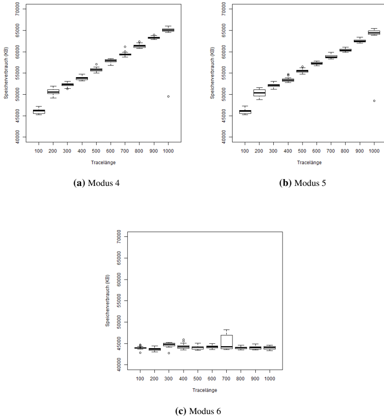
Abbildung 7.6: Speicherbedarf des ProSP in Abhängigkeit von der Tracelänge (10 personenbezogene Daten, 100 KB Dateien)
