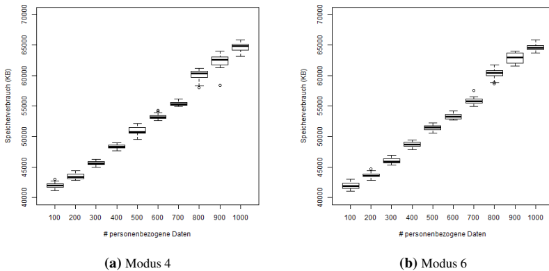
Abbildung 7.5: Speicherbedarf des PIP in Abhängigkeit von der Anzahl der personenbezogenen Daten (Tracelänge 100, 100 KB Dateien)
