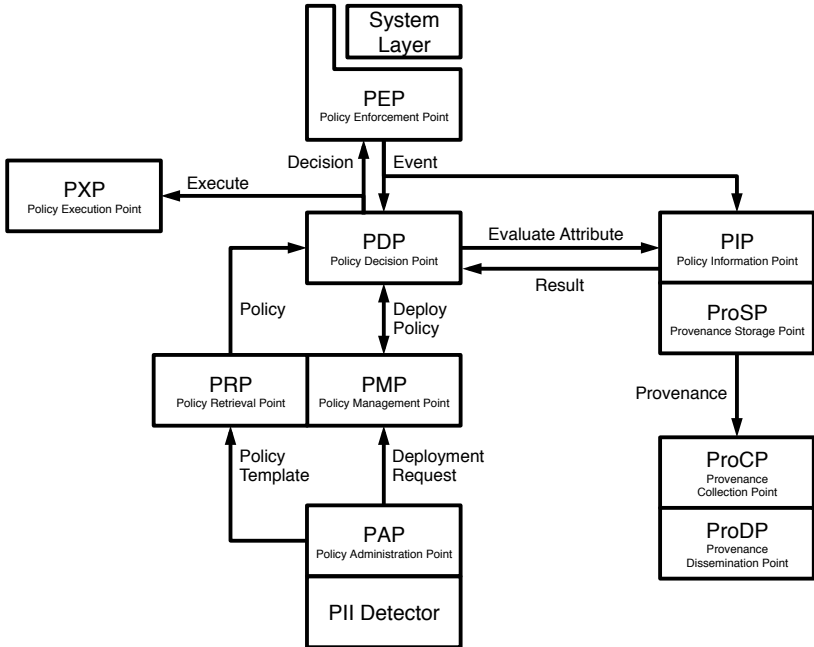
Abbildung 5.3: Logische Usage-Control- und Provenance-Architektur
