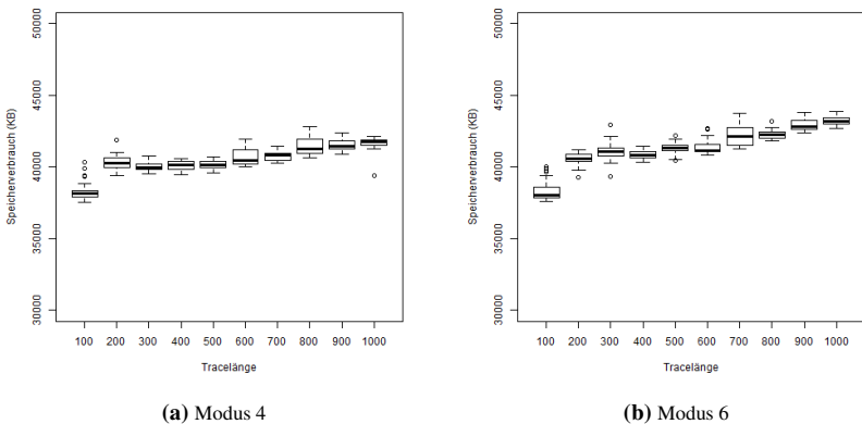
Abbildung 7.4: Speicherbedarf des PIP in Abhängigkeit von der Tracelänge (10 personenbezogene Daten, 100 KB Dateien)
