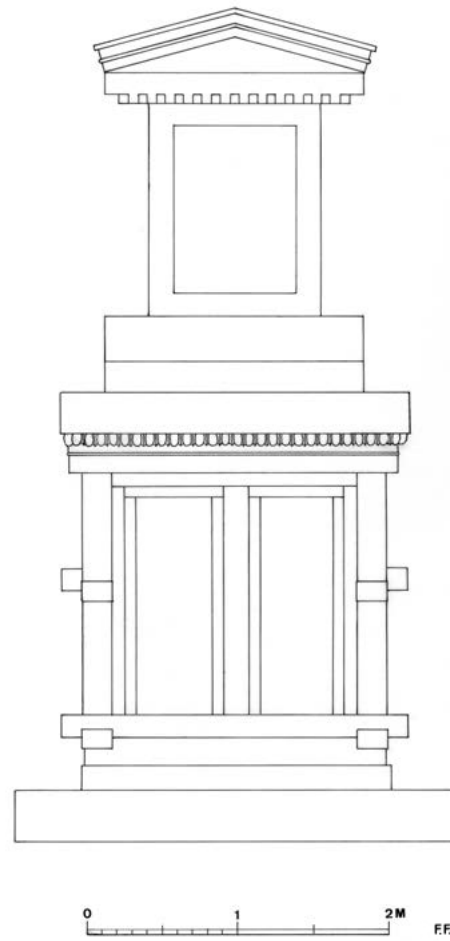
2. Rekonstruktion des Grabbaus (2)
