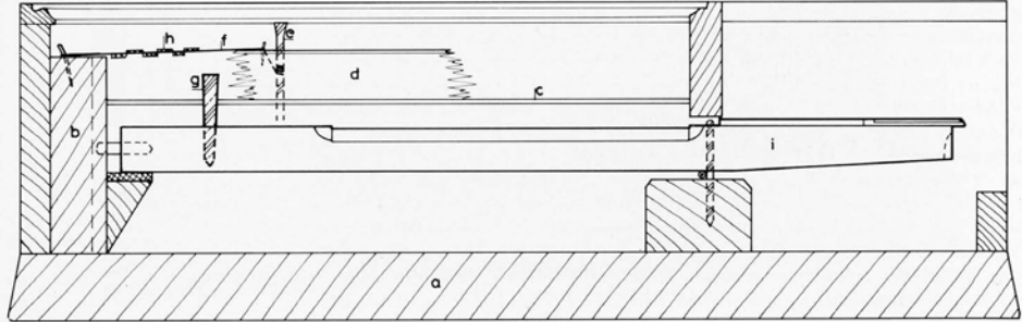
Mechanik-Modell des niederländischen Klavichords
