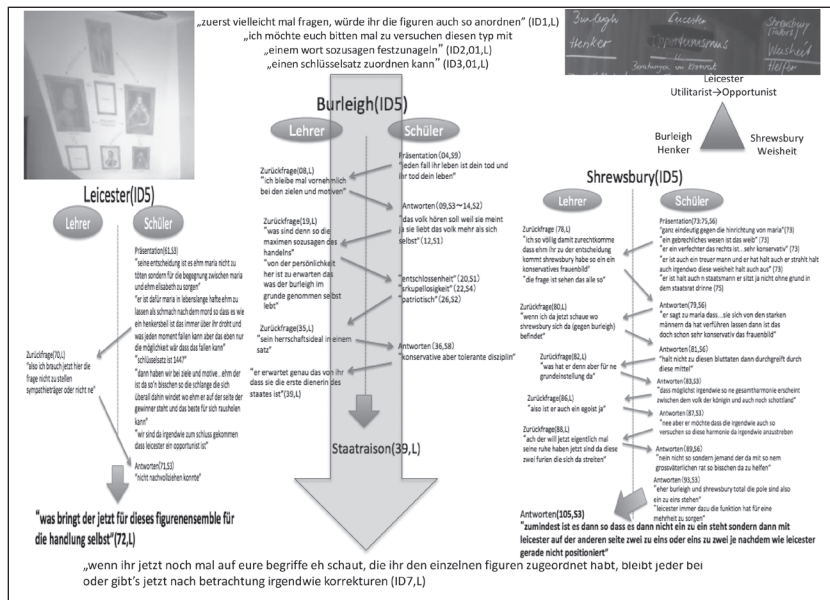
Abb. 1: Unterrichtsstruktur
