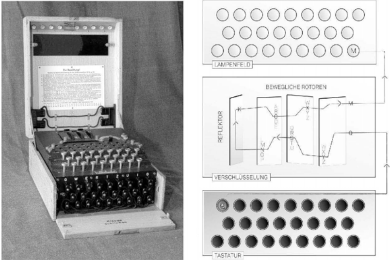
Chiffriermaschine Enigma und schematische Darstellung. (Foto D.Landwehr; Schema I. Sterzinger)
