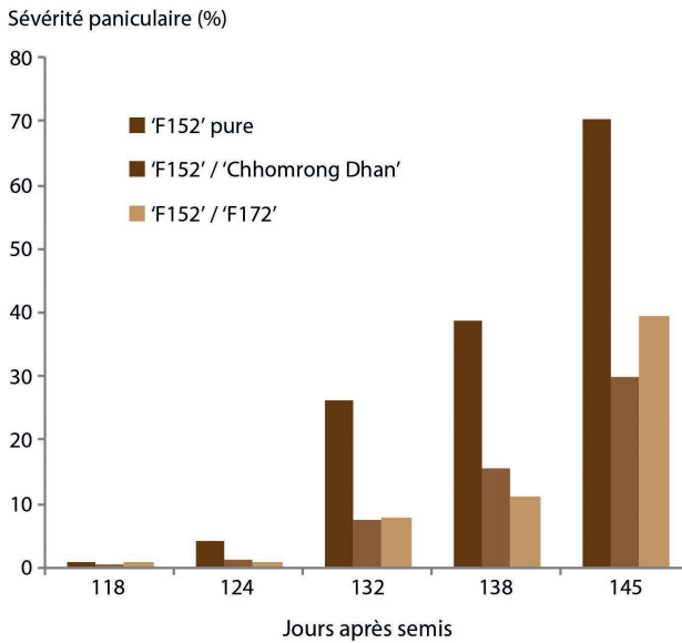
Figure 2.5b. Évolution du pourcentage de grains atteints par la pyriculariose sur la variété 'F152' (sensible) cultivée pure ou en mélange (une ligne de sensible pour quatre lignes de résistantes) avec les variétés 'Chhomrong Dhan' (tolérante) ou 'F172' (résistante), en 2012.
