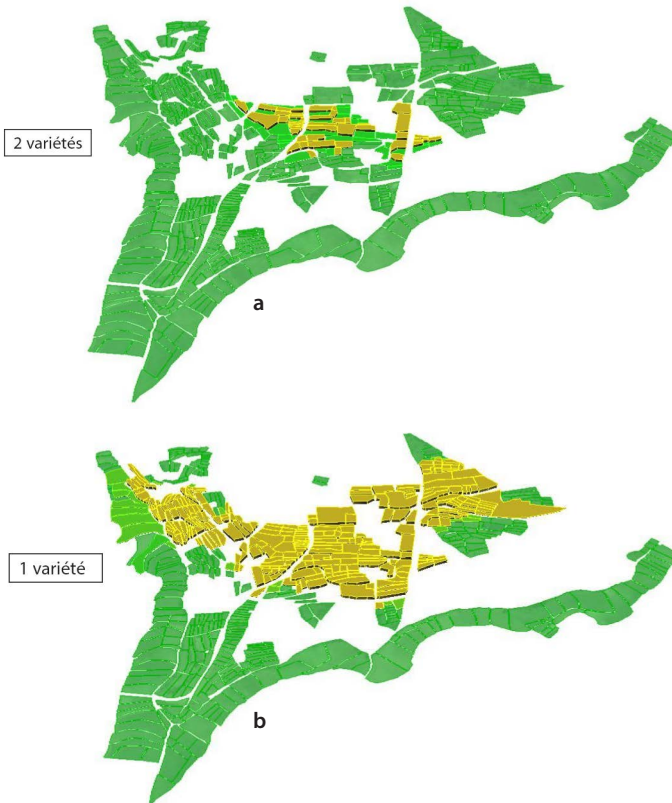
Figure 2.6. Simulations de cinq ans de l'attaque de pyriculariose sur un paysage agricole malgache dans lequel toutes les parcelles sont cultivées en riz chaque année. (a). Une variété en rizière et deux variétés en pluvial. (b) Une variété en rizière et une variété en pluvial. L'infestation initiale est identique dans les deux cas. La hauteur des pavés colorés est proportionnelle au niveau d'attaque par la maladie.
