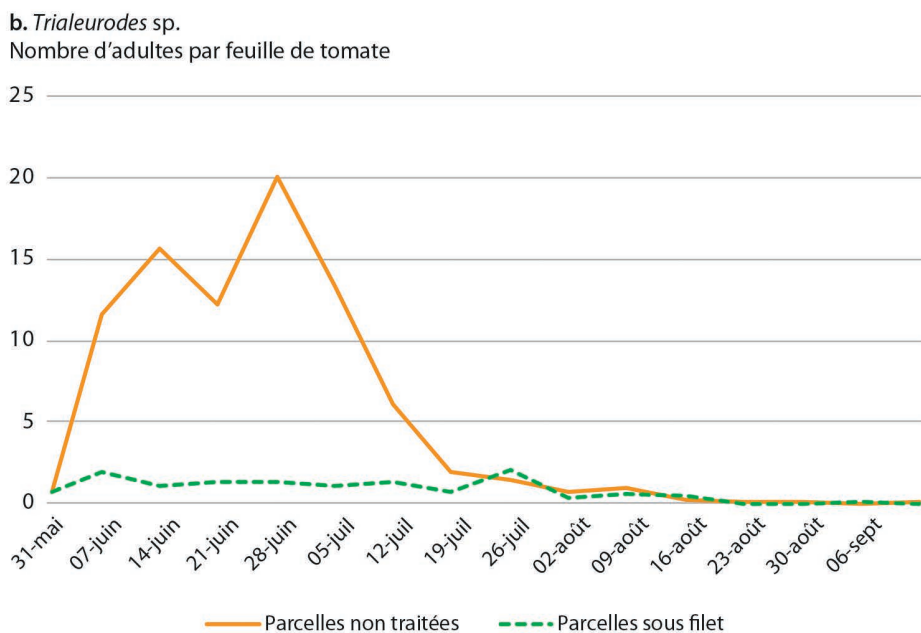
Figure 4.1. Nombre moyen de Tuta absoluta (a) et de mouches blanches Trialeurodes sp. (b) par feuille de tomate non traitée, sous filet (trait pointillé) et hors filet (trait plein), dans une expérimentation conduite au Kenya en 2017 sur la station du Kalro, à Mwea.
