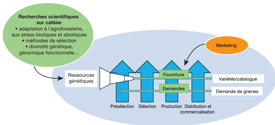
Figure 9.4. Processus de création variétale chez Coffea arabica pour l'adaptation à l'agroforesterie et aux changements climatiques.
