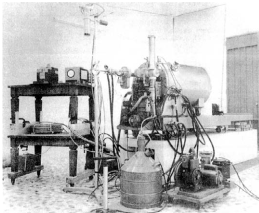
Figura 28 – L'acceleratore PN400 della High Voltage Engineering Co. e i suoi servizi, installato nel bunker di Arcetri. L'acceleratore è ora esposto nell'atrio del Dipartimento di Fisica e Astronomia a Sesto Fiorentino. [Taccetti 2017]
