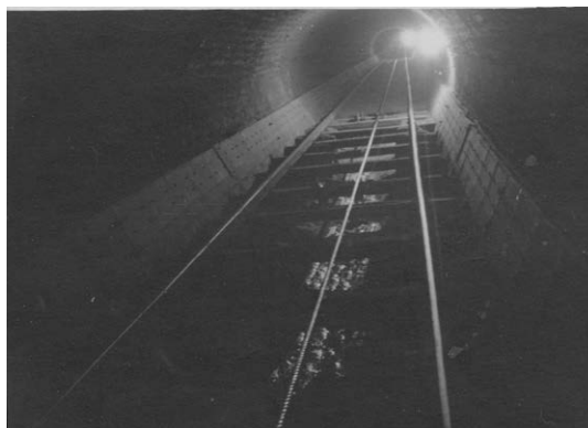
Figura 25 – 1940: Il pozzo della galleria direttissima dove fu eseguito l'esperimento di Ballario, Della Corte e Prosperi. [Fondo Della Corte, Biblioteca di Scienze, Università di Firenze]
