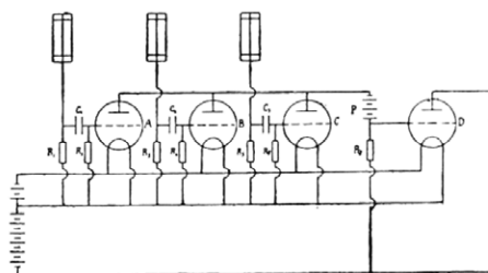
Figura 17 – Il circuito di Rossi per rivelare coincidenze di raggi cosmici che arrivano sui contatori Geiger (i rettangoli in alto dello schema). [Rossi 1930]
