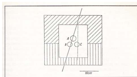
Figura 18 – L’uso del circuito di Rossi per rivelare una coincidenza tripla che, nella disposizione in figura dei tre contatori, mostra la produzione di una radiazione secondaria (linea tratteggiata) da parte della radiazione primaria (linea continua). [Rossi 1932]
