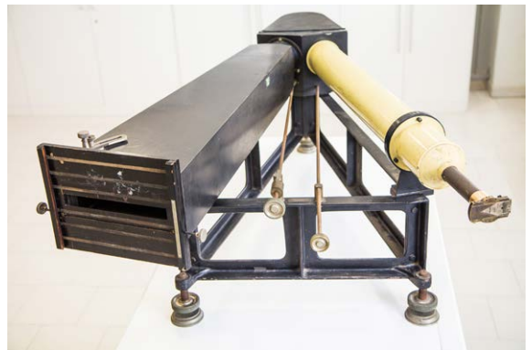
Figura 8 – Spettrografo a reticolo progettato da Rasetti (1925 circa) e fatto costruire alle Officine Archimede di Firenze. Rasetti non ebbe mai la possibilità di utilizzare lo strumento per risultati pubblicabili, perché nel 1927 si trasferì a Roma a lavorare con Enrico Fermi, con il quale pubblicò immediatamente (1927, 1928) lavori di spettroscopia eseguiti con uno spettrografo a grande braccio presente a Roma. Alla fine del 1965 questo strumento fu portato nei laboratori di spettroscopia del Centro Microonde del CNR in Firenze e ivi utilizzato per eseguire il primo esperimento di spettroscopia non-lineare eseguito in Italia. [Dipartimento di Fisica e Astronomia, Università di Firenze, foto di R. Baglioni]
