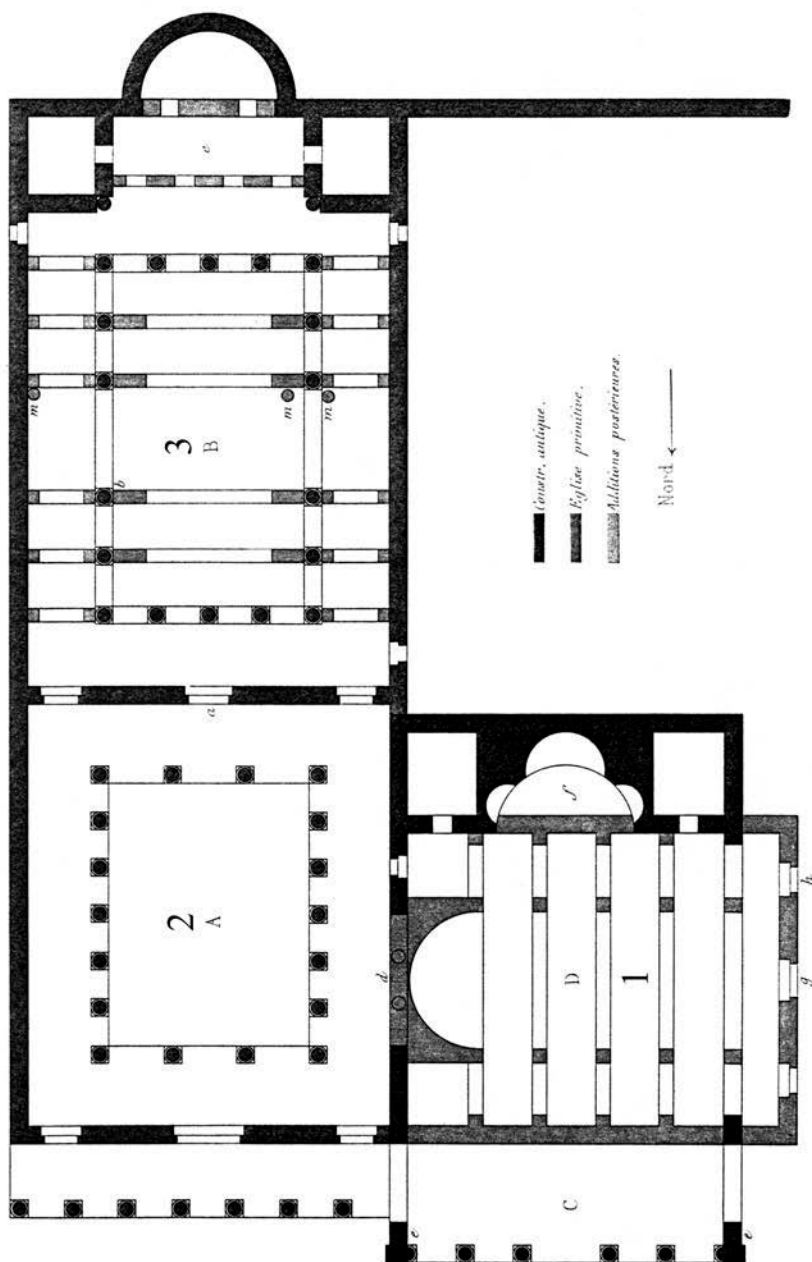
Abb. 6a: Kanatha, „Serail“, 1 = „Westtempel“, 2 = Hof, 3 = „Osttempel“; a: Grundriss nach Vogüé
