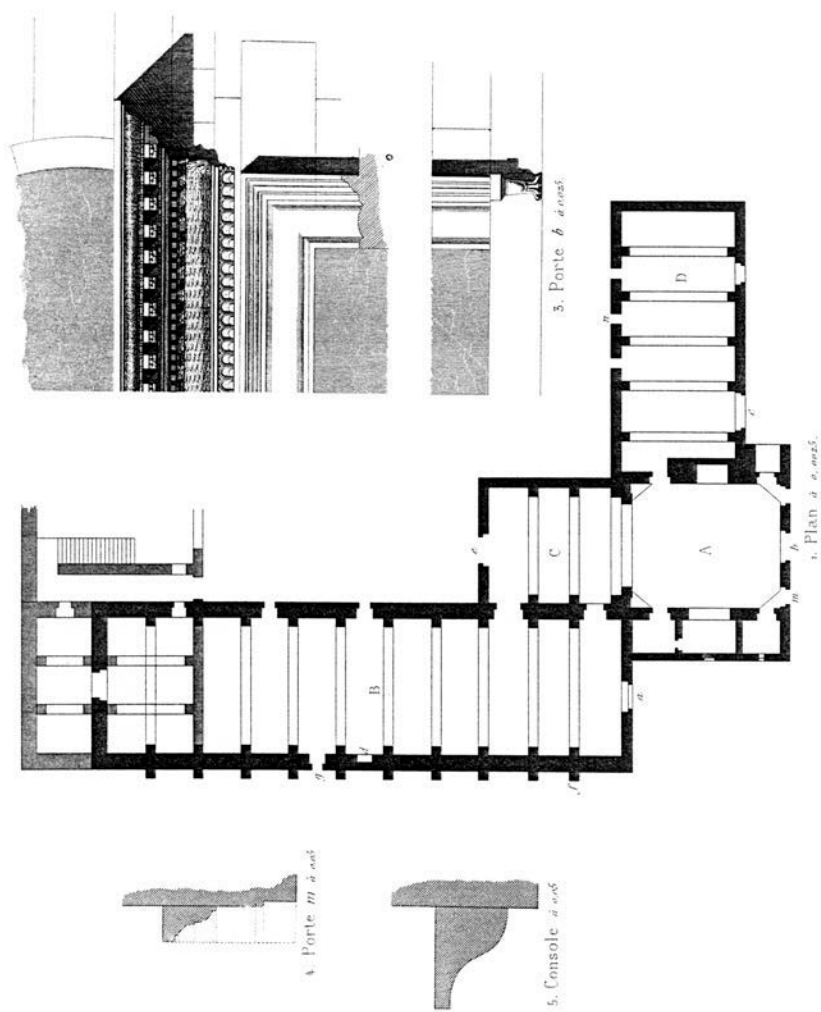
Abb. 16a: Shaqqa, „Kaisariye“; a: Grundriss nach Vocüé
