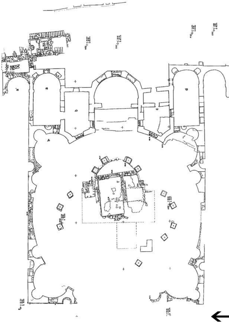
Abb. 10: Bostra, Kirche des Sergios, Bacchos und Leontinos, Grundriss.
