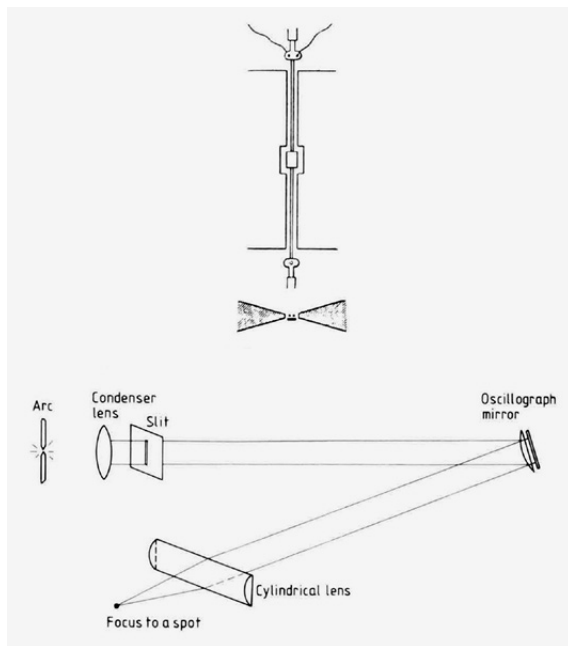
22 Schleifenoszillograf, 1893
