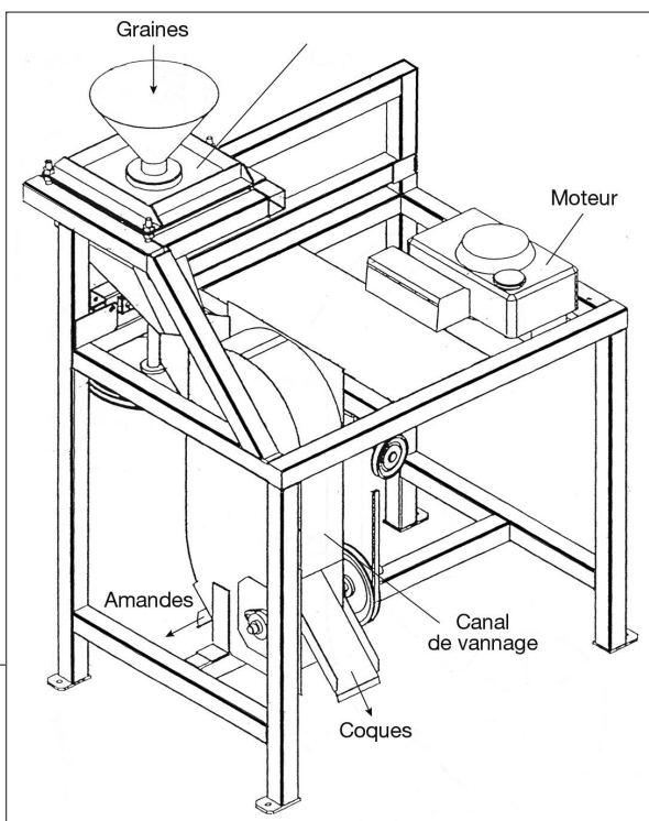
Figure 4.16.2. Vue d'ensemble du décortiqueur à néré (© Patrice Thauay, Cirad).
