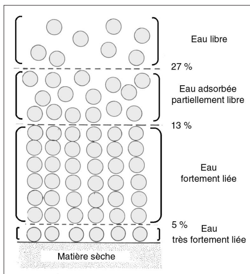
Figure 2.4. Schéma de fixation de l'eau dans un grain de céréale (d'après Lasseran, 1977).
