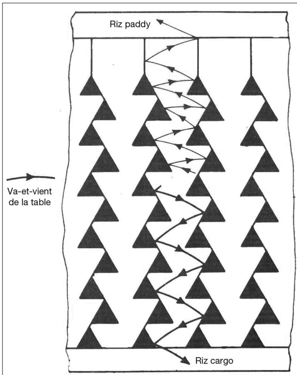
Figure 3.14. Schéma de séparation du riz paddy et du riz cargo (d'après Gariboldi, 1974).
