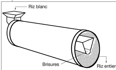
Figure 3.19. Schéma du trieur à alvéoles (d'après Borasio et Gariboldi, 1957).
