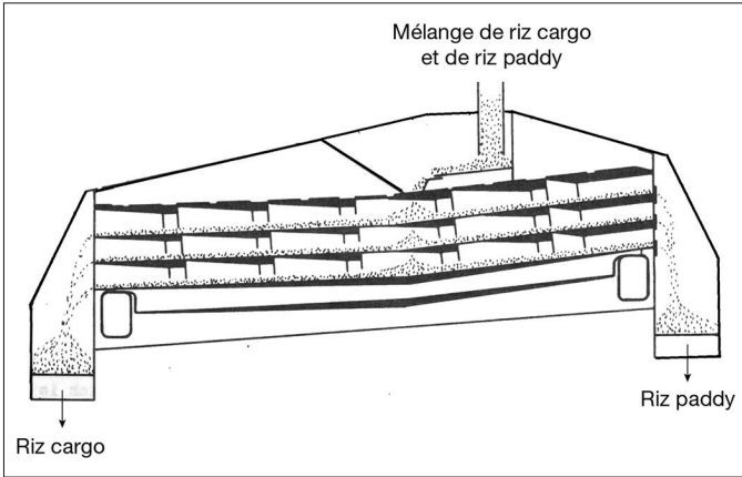
Figure 3.13. Table densimétrique à trois étages (d'après Gariboldi, 1982).
