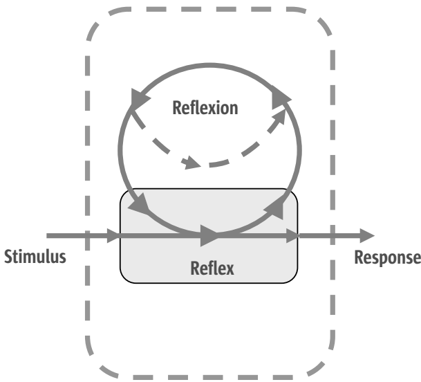
Abb. 4 Das Bedingungsgefüge von reflexartigem und reflektiertem Verhalten.
